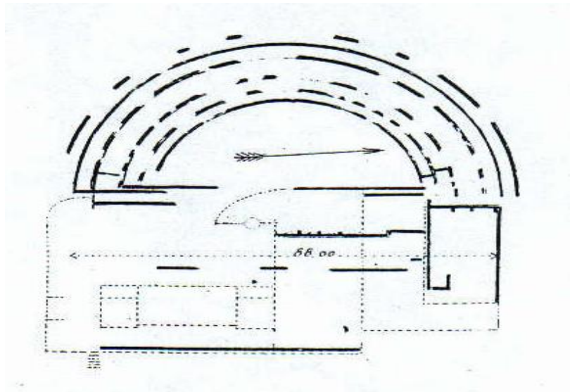
(الشكل 57) مسرح روسيكاد Théâtre de RUSICADE
