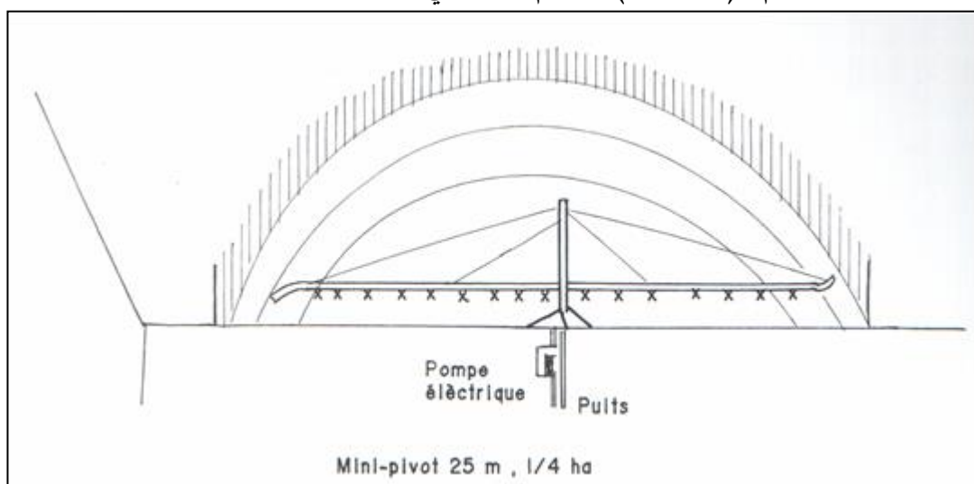
لشكل رقم: (03-09) : رسم تخطيطي للرش المحور المصغر.
