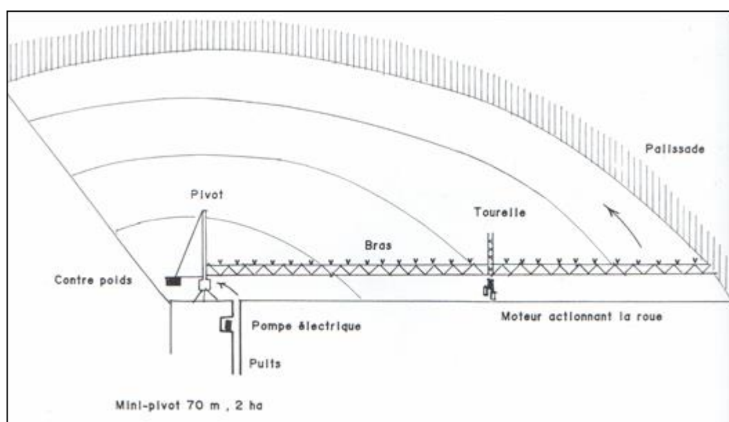
الشكل رقم: (03-10): رسم تخطيطي للرش المحور PIV
