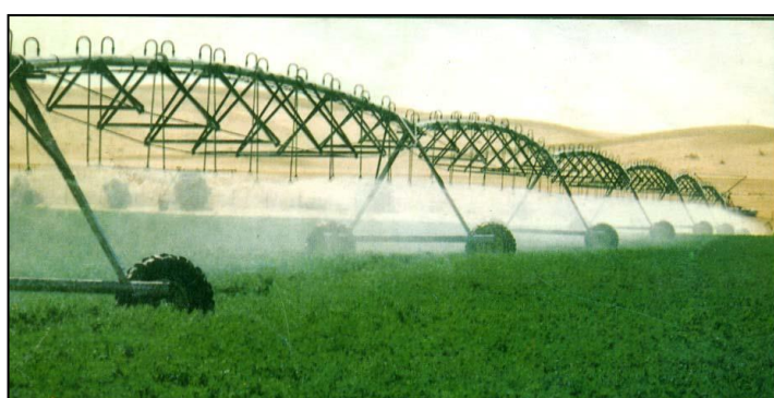
الرش المحور الأمريكي بطول 500 م
