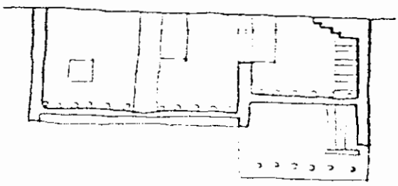
Coupe XX
