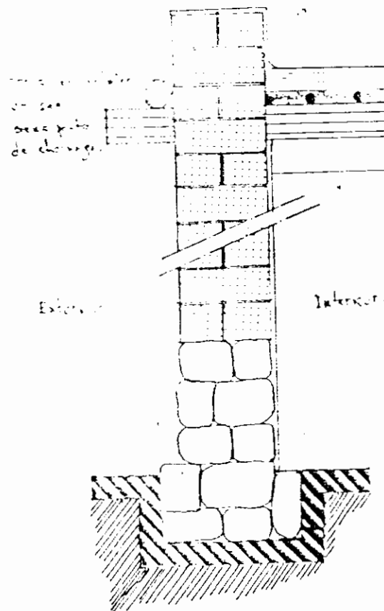
Coupe sur le mur
