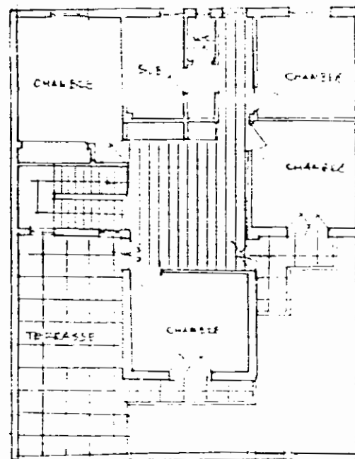
Plan étage
