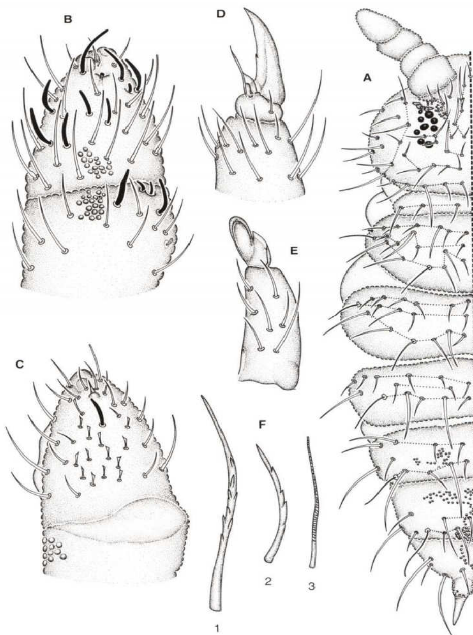
Fig. 30 : Ceratophysella gibbosa Bagnall, 1940.
