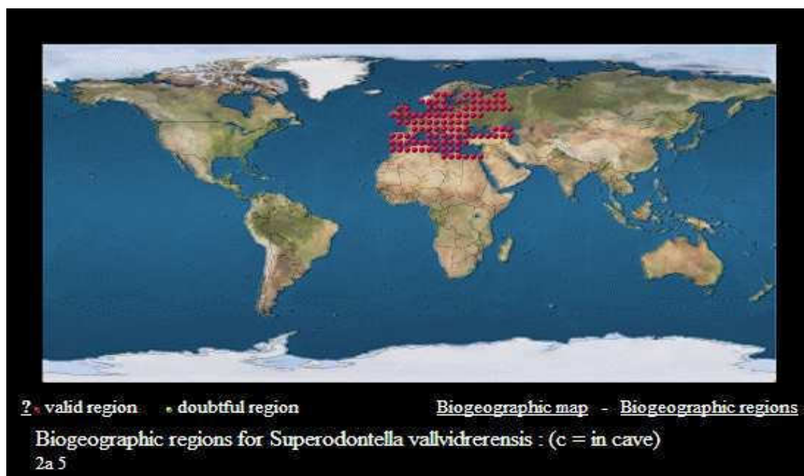
Fig.57: Aire de répartition biogéographique de Superodontella vallviderensis : euro-méditerranéennes. (Bellinger & al, 2014)
