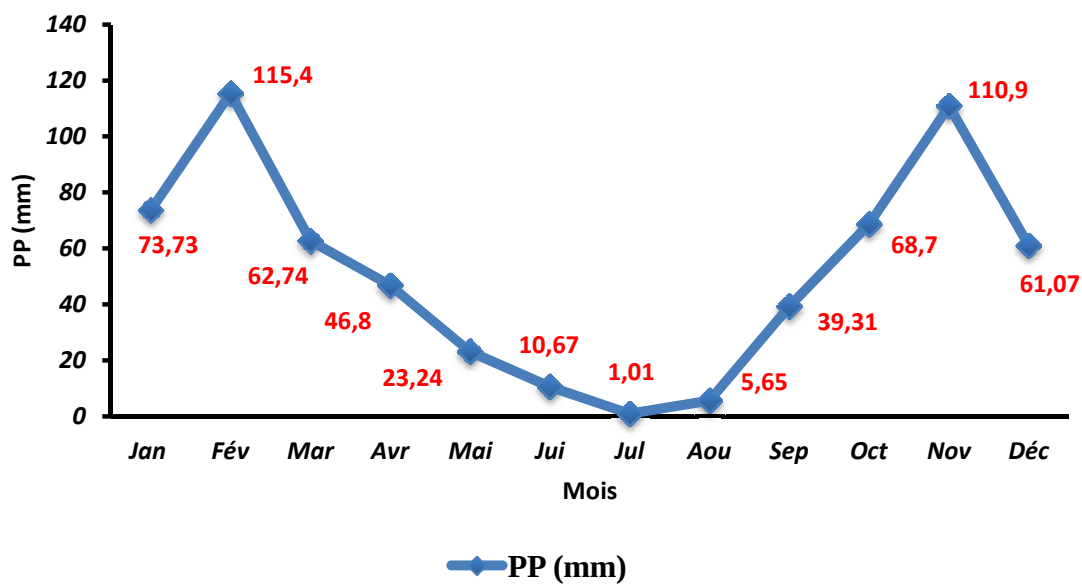
Fig.17 : Variation des précipitations moyennes mensuelles de 2010 à 2013 pour la région d'Annaba.
