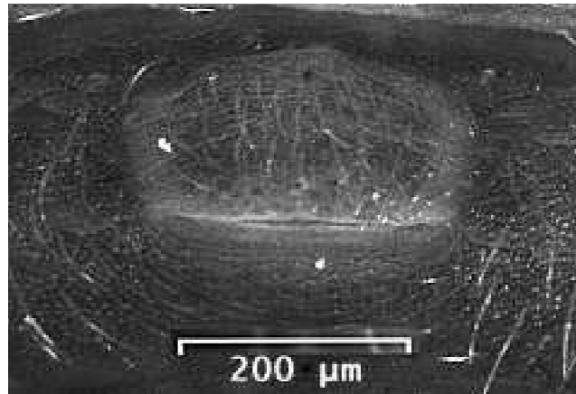
Fig. 7 (b): Orifice génital femelle chez Tetrodontophora bielanensis (Bellinger & al., 2014)
