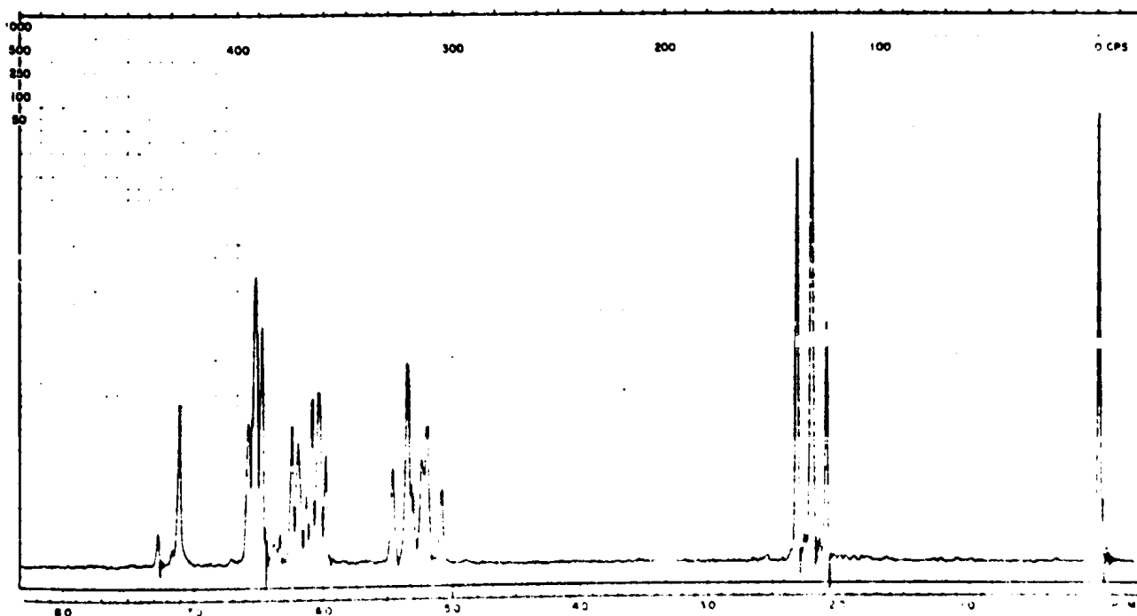
Fig. III,1 : Spectre R.M.N. du tropilidène
