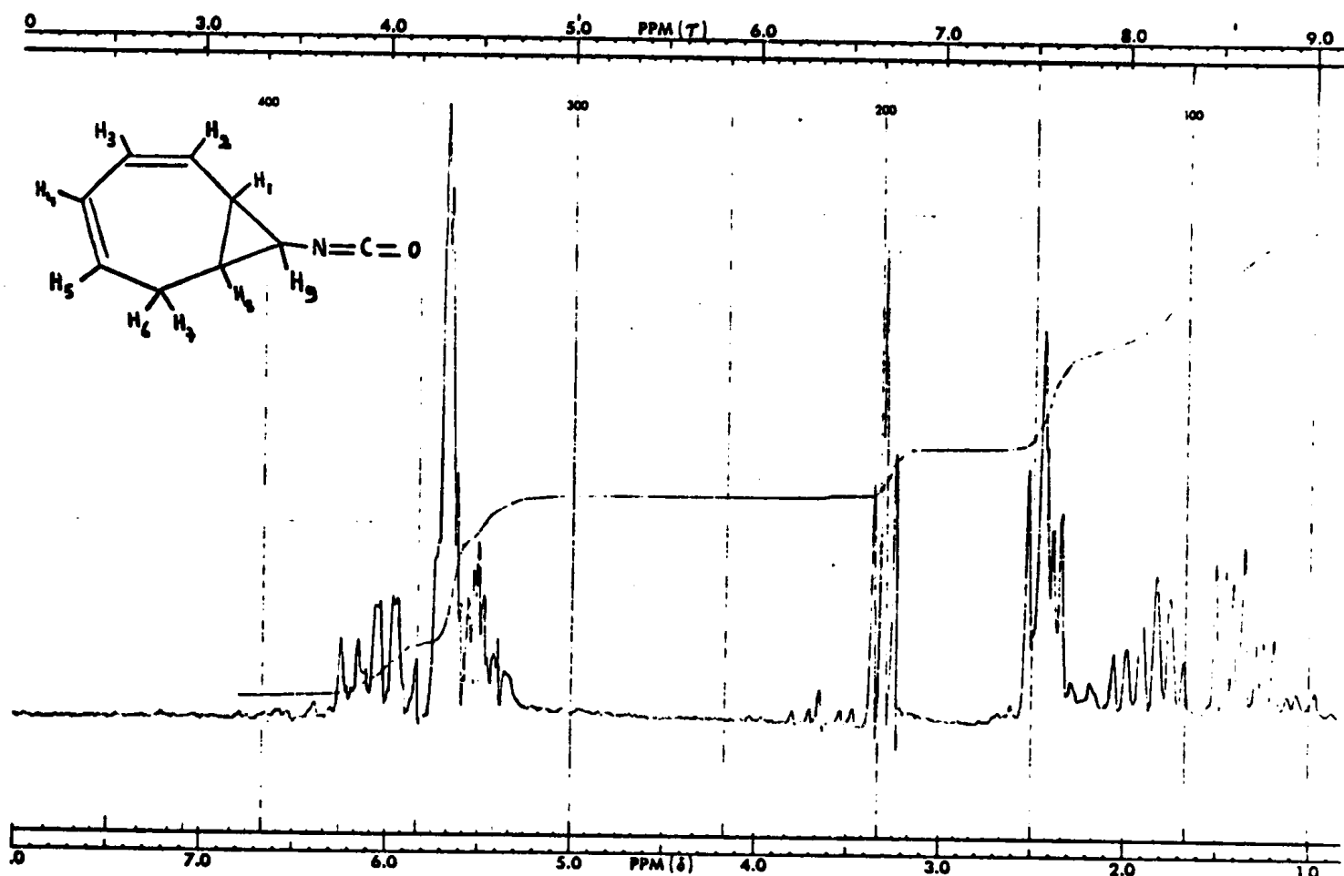
Fig. I,3 : Spectre RMN du bicyclo (5,1,0) octadiène-2,4 yl-8 isocyanate
