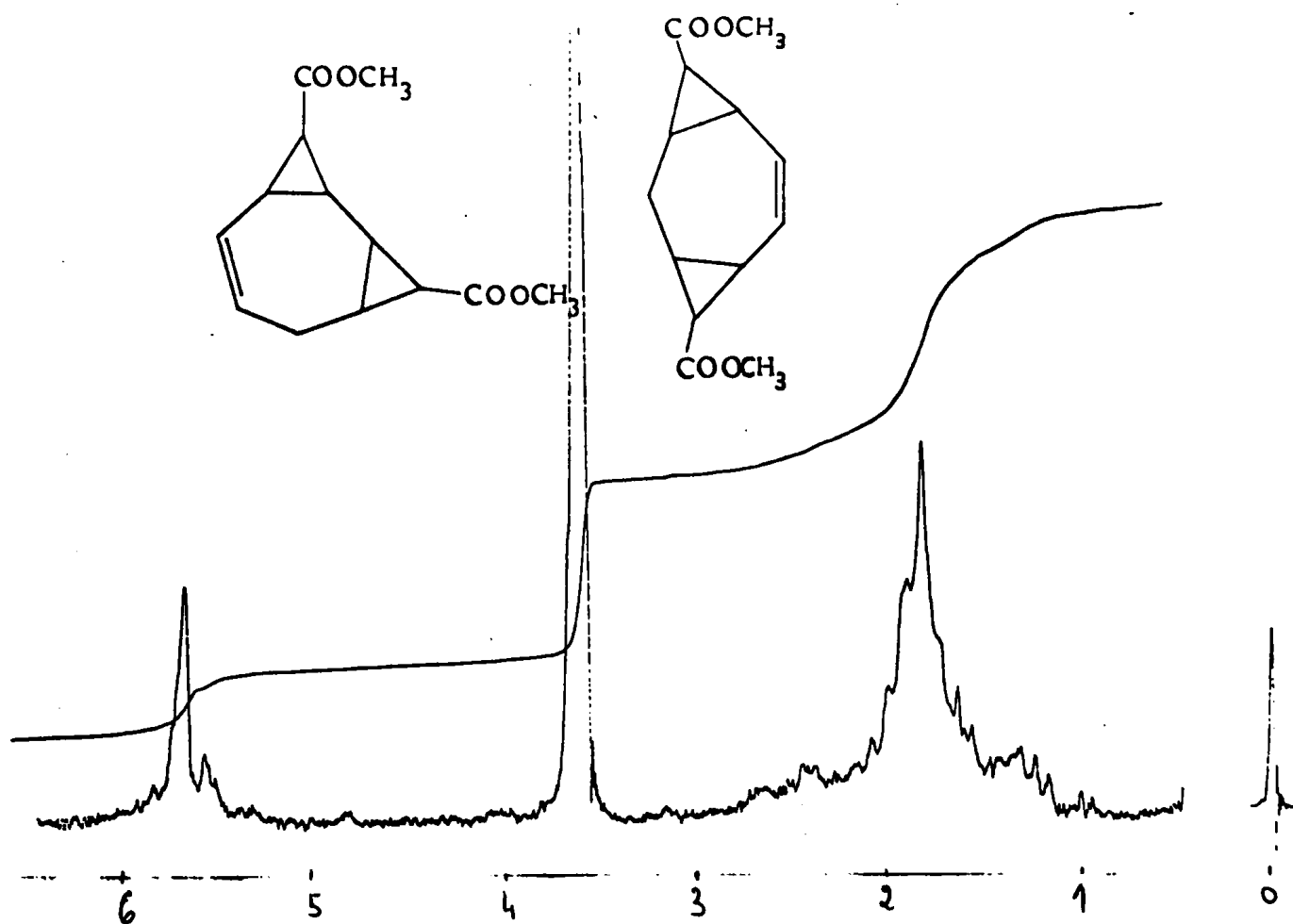
Fig. I,6 - Spectre RMN du diester tricyclique 2 .
