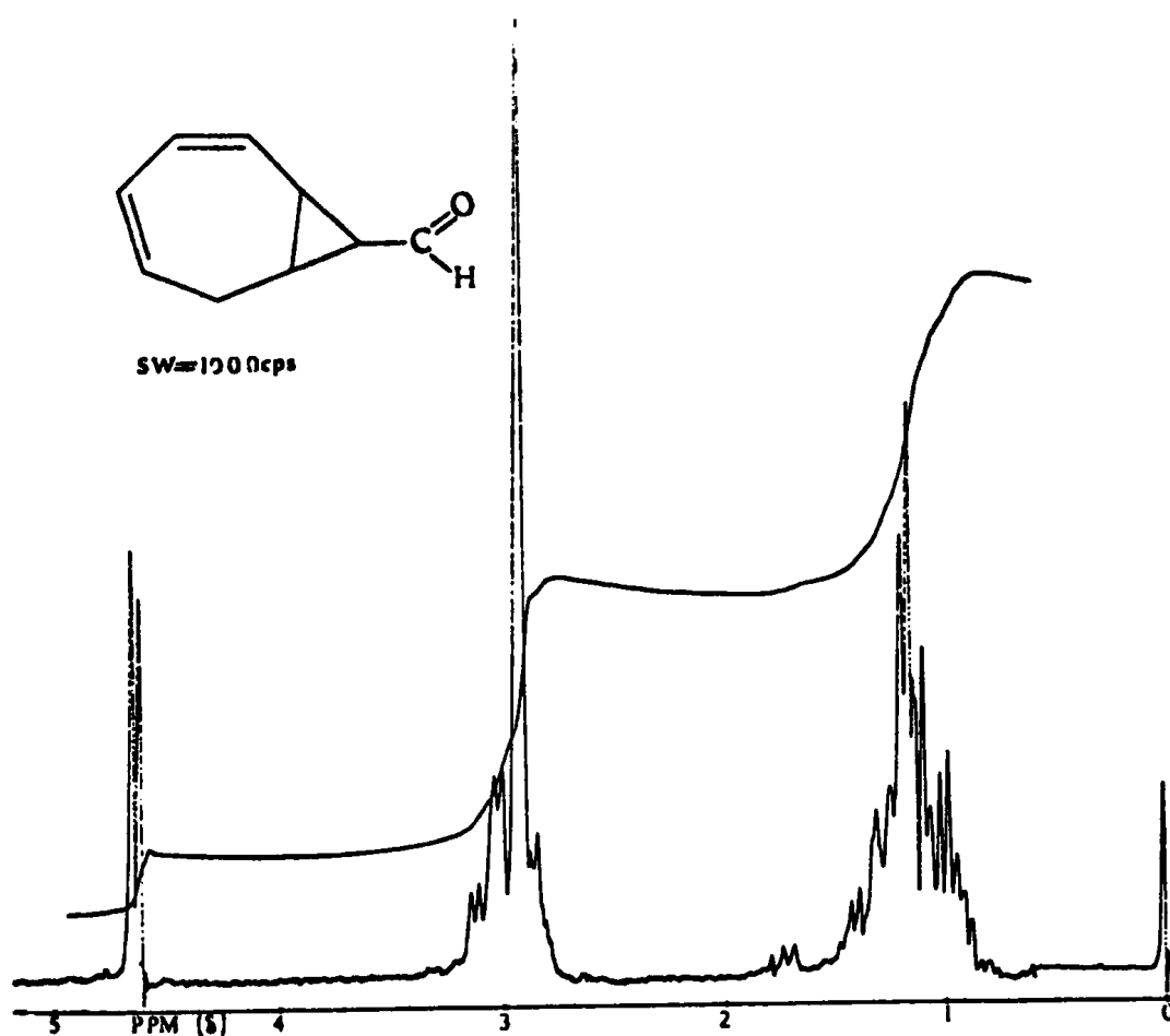
Fig.VI,1 Spectre RMN du bicyclo (5,1,0) octadiène-2,4 yl-8 carboxaldéhyde.
