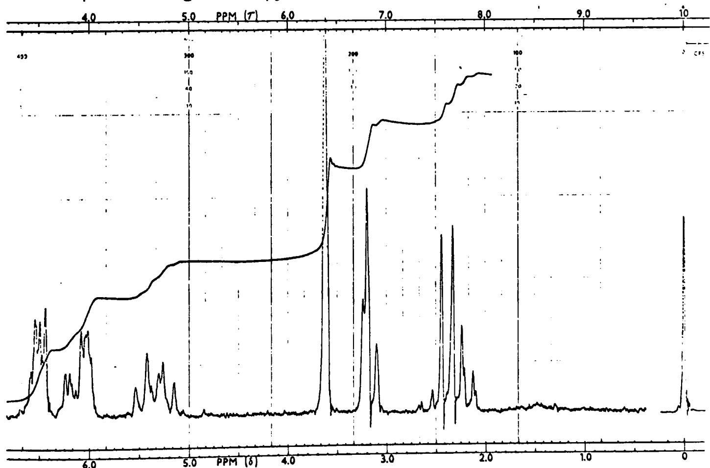
Fig. IV,4 Spectre RMN du mélange des tropyl-1,2,3 acétate de méthyle obtenu par chauffage du tropyl-7 acétate de méthyle 6h à 200°C.
