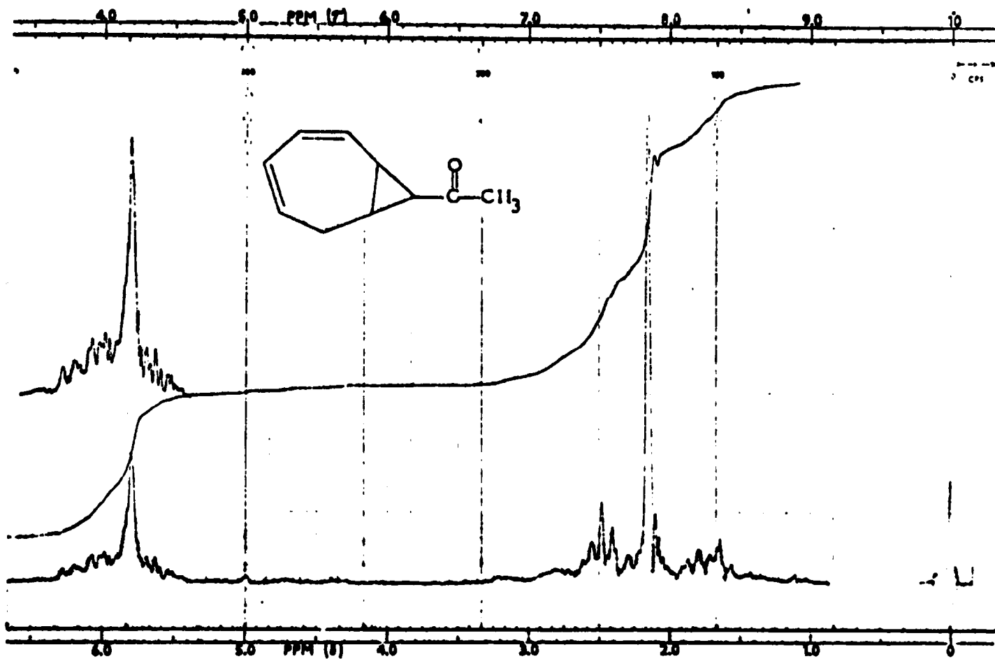
Fig. II,2 - Spectre RMN de la bicyclo (5,1,0) octadiène-2,4 yl-8 méthyl cétone
