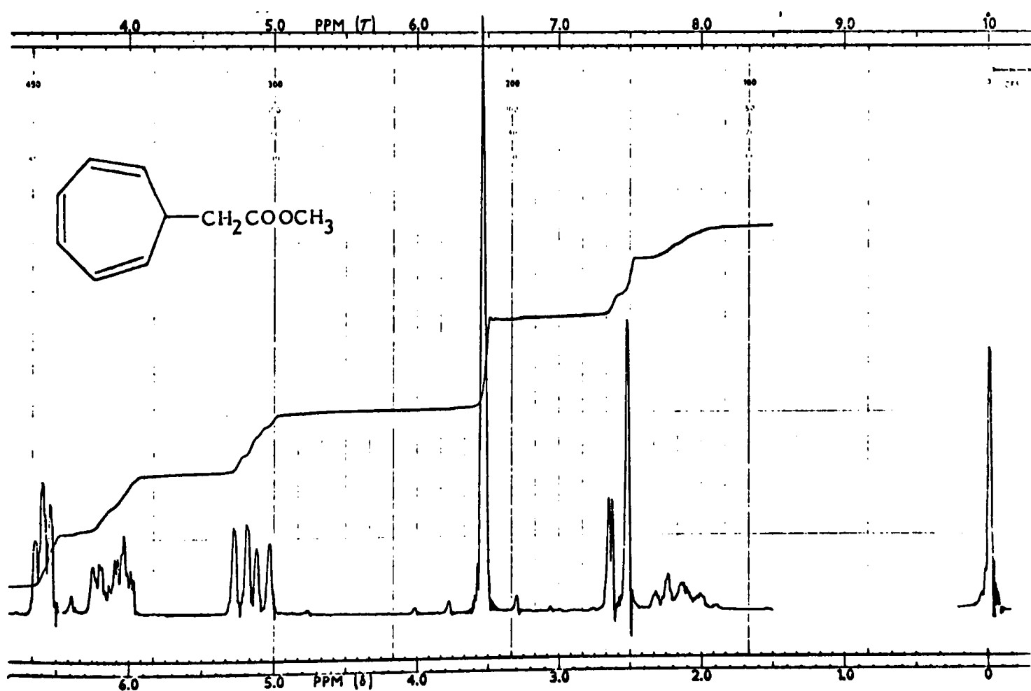
Fig. IV,2 Spectre RMN du troyl-7 acétate de méthyle
