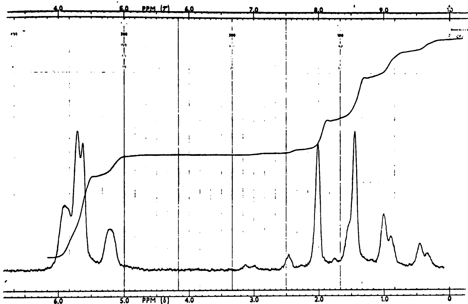
Fig. IV,5 Etallement de la région méthylénique de la figure IV,4 ( SW = 100cps )
