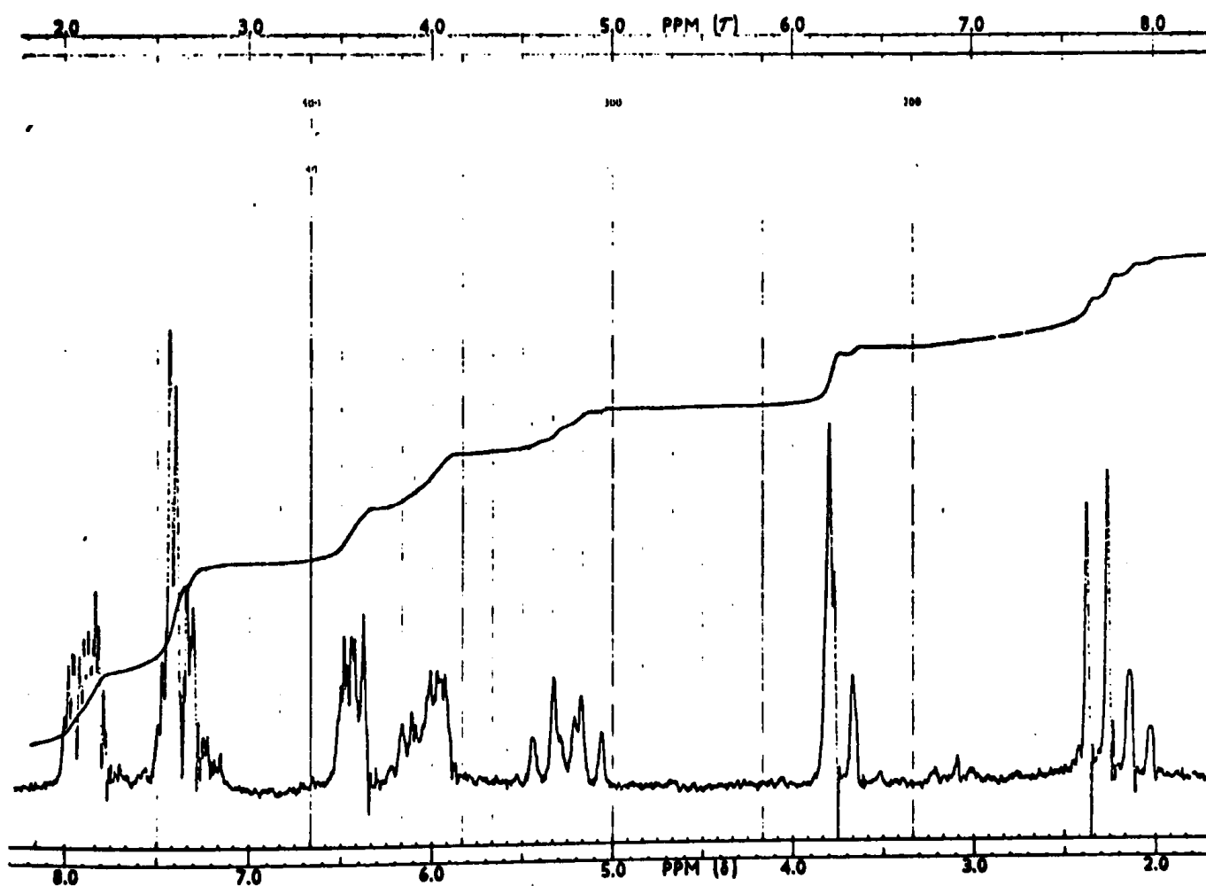
Fig. IV,6 Spectre RMN du mélange des troyl-1,-2,-3 acétophénones
