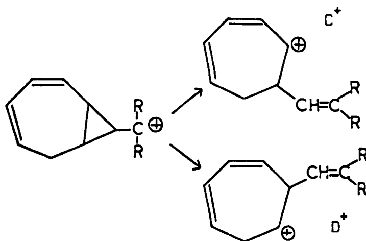
Fig.III,6 Intermédiaires pouvant se former lors de la déshydratation des alcools.
