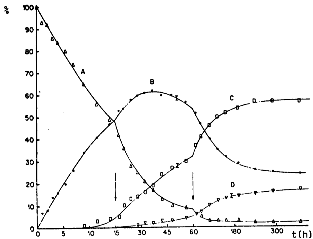
Fig. IV,1 Pourcentage des isomères formés à partir du méthyl-7 tropilidène en fonction du temps à 140°C
