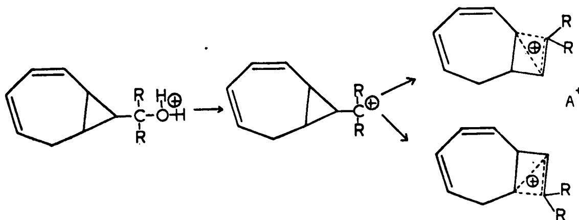
Fig. III,5 Cations intermédiaires pouvant se former lors de la déshydratation des alcools.
