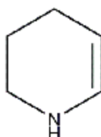
3- Azacyclohexène
