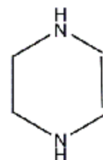
3, 6- Azacyclohexène
