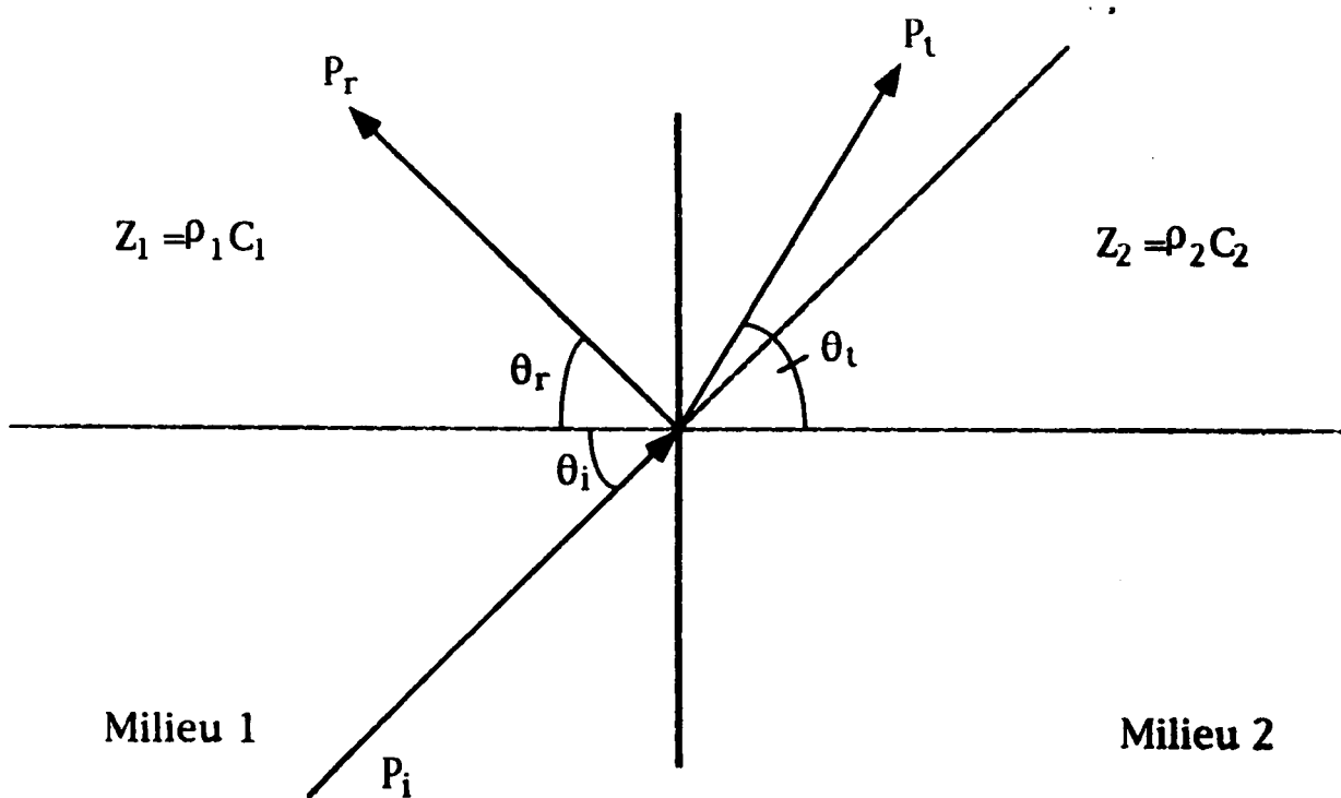
Fig (5.3): Incidence oblique d'une onde acoustique cas où C_1 < C_2
