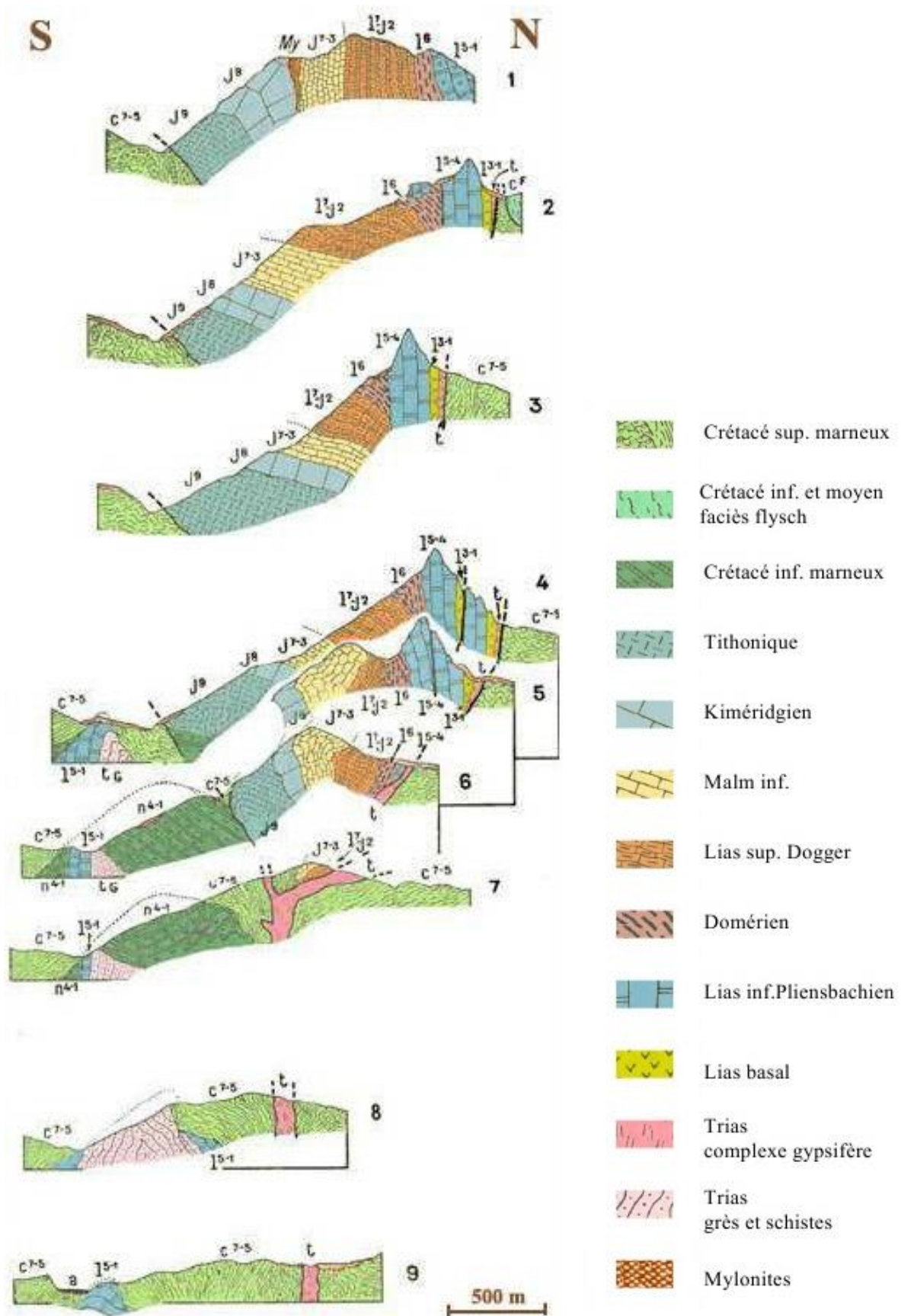
Figure 10: Coupes séries du Djebel Sidi Maarouf (Durand Delga, 1955).
