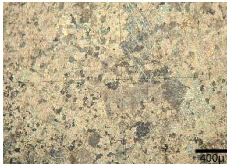
Figure 38: Dolomie à cristaux relativement fins.
