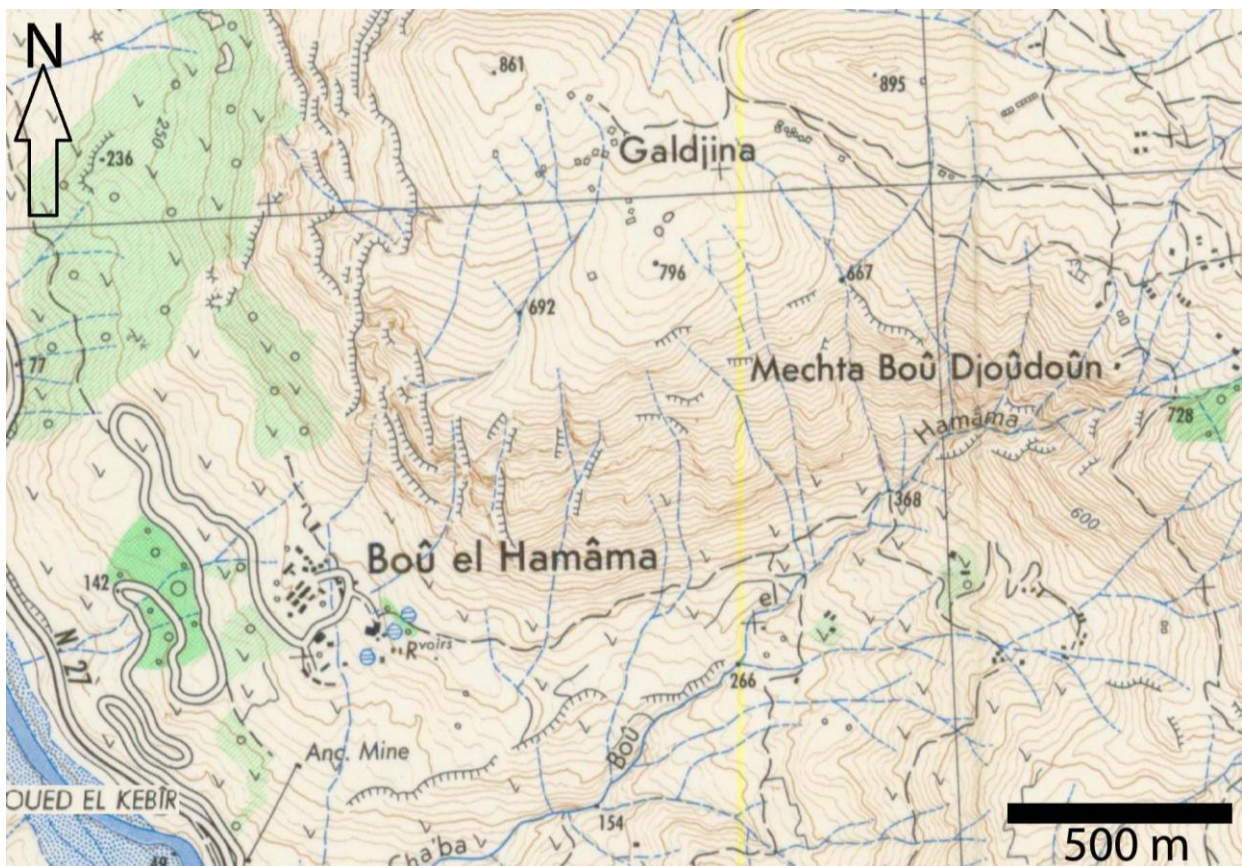
Figure 03: Situation géographique de Kef Boulehmane (Extrait de la carte topographique d'Ain Kechera au 25.000°).
