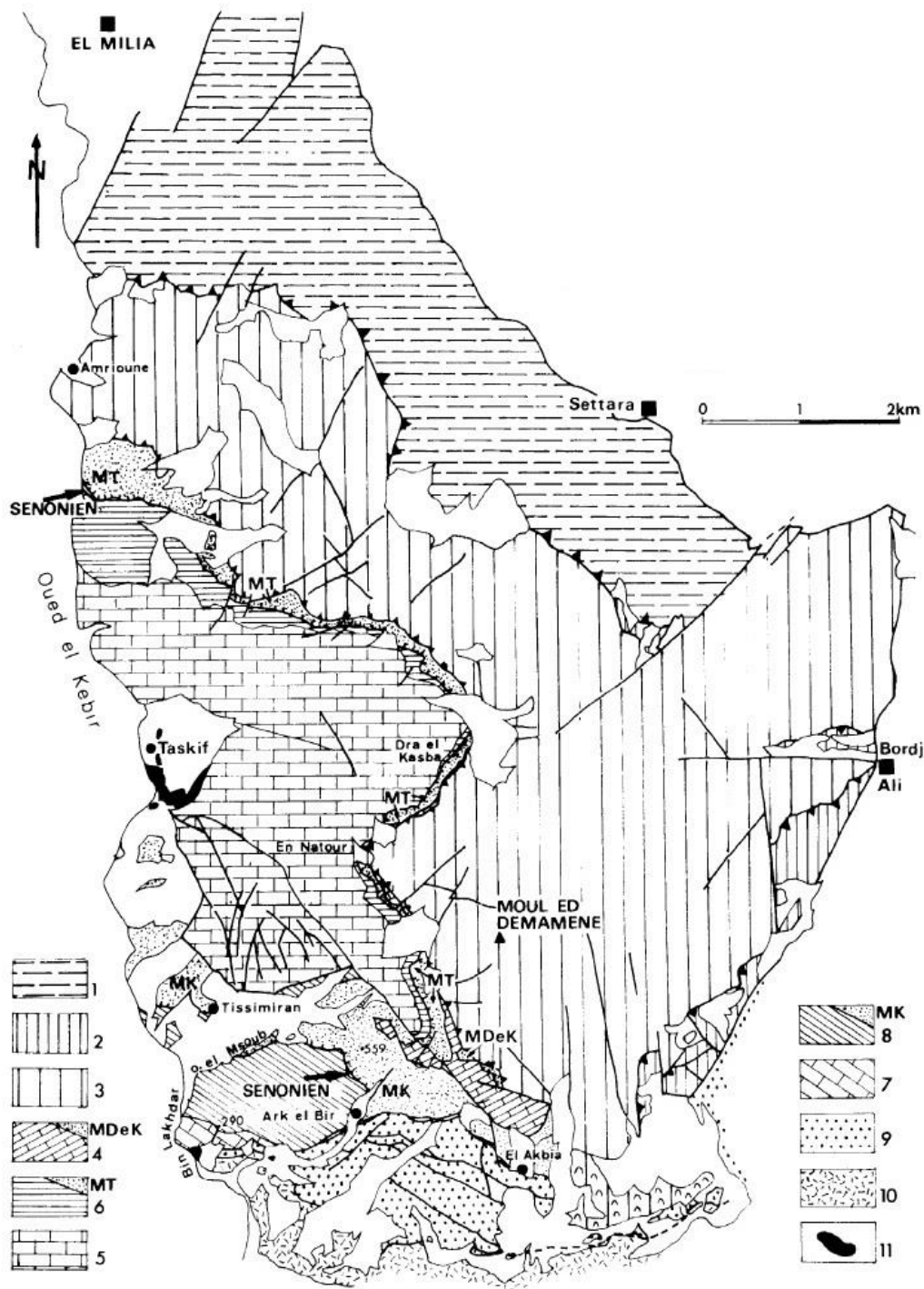
Figure 20: Carte simplifiée des écaïlles inférieures de Moul ed Demamène dans leur cadre structural (Bouillin, 1977).
