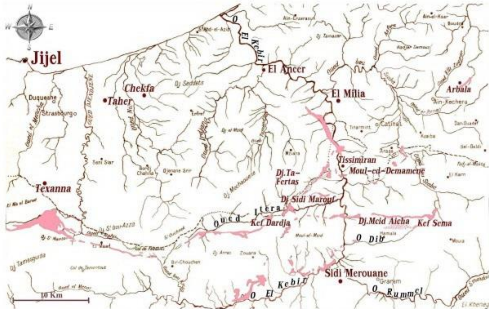
Figure 09: Répartition géographique des affleurements du Trias (Durand Delga, 1955).
