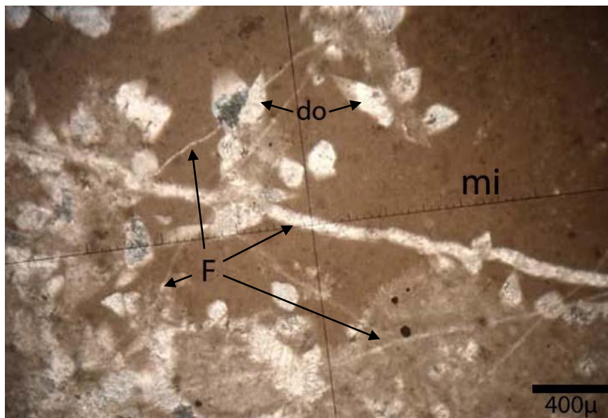
Figure 36: Photo montrant le phénomène de dolomitisation dans un calcaire micritique (do, dolomites ; mi, micrite ; F, micro-fractures en « scheet cracks »).
