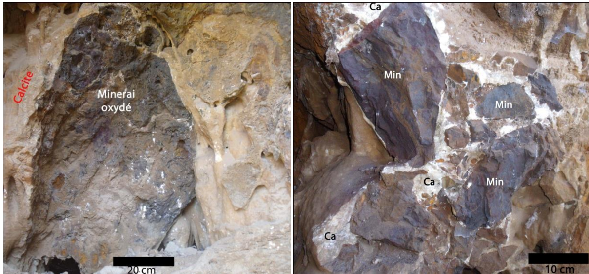
Figure 62: La disposition des éléments oxydés de taille distincte avec la calcite à l'entrée de la galerie (Min, Mineral ; Ca, Calcite).
