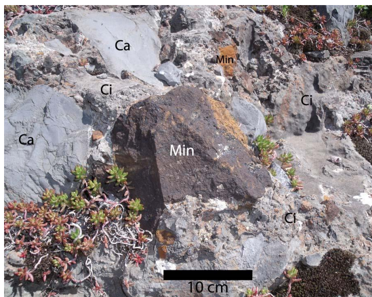
Figure 63: Brèche polygénique à éléments de différente taille, et à ciment carbonaté (Min, Mineral ; Ca, Calcaire ; Ci, Ciment).
