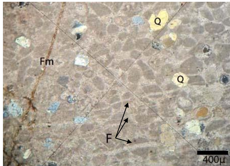
Figure 44: Micro-fractures (F) remplies par la sparite (Fm, micro-fracture oxydée).
