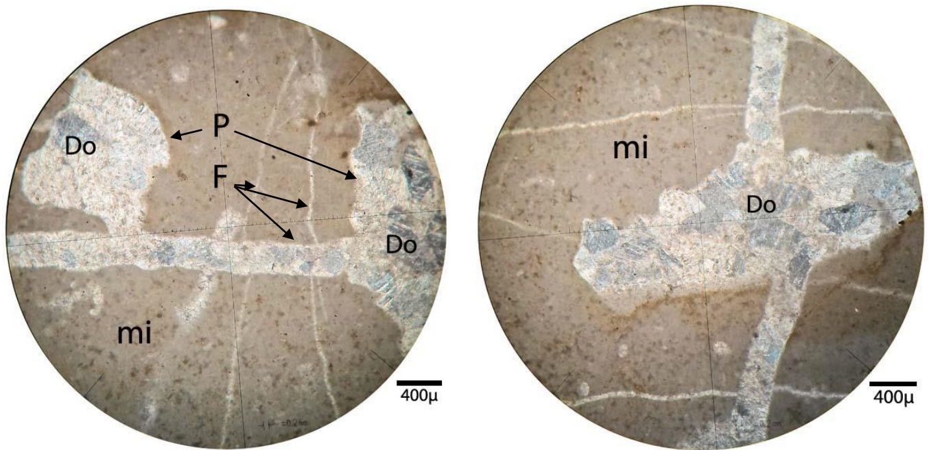
Figure 37: Photos, illustrant des fronts de remplacement de la micrite par de la dolomite et/ou calcite. Dolomite et/ou calcite (Do) ; micrite (mi) ; fractures (F) ; poches (P).
