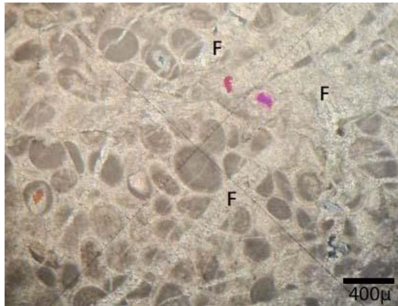
Figure 41: Remplissage des fractures par la calcite de recrystallisation.
