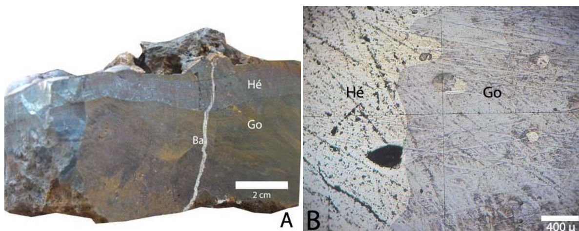
Figure 29: Photos macro (A) et microscopique (B), montrant l'association hématite (Hé)-goethite (Go) et barytine (Ba).
