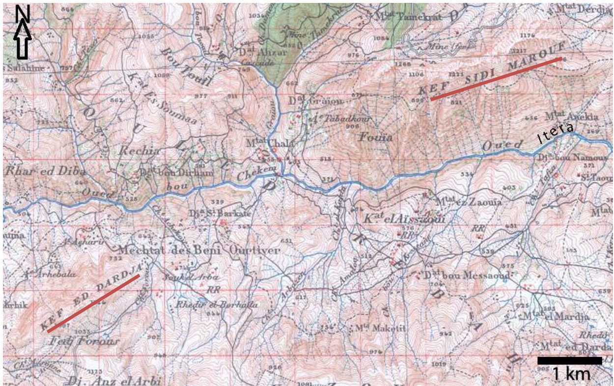
Figure 02: Situation géographique de Kef Sidi Marouf et Kef Dardja sur la carte topographique de Sidi Merouane au 50.000°.
