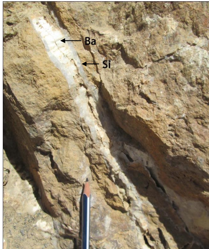
Figure 45: Photo illustrant le remplissage d'une fracture par la silice (Si) et la barytine (Ba).
