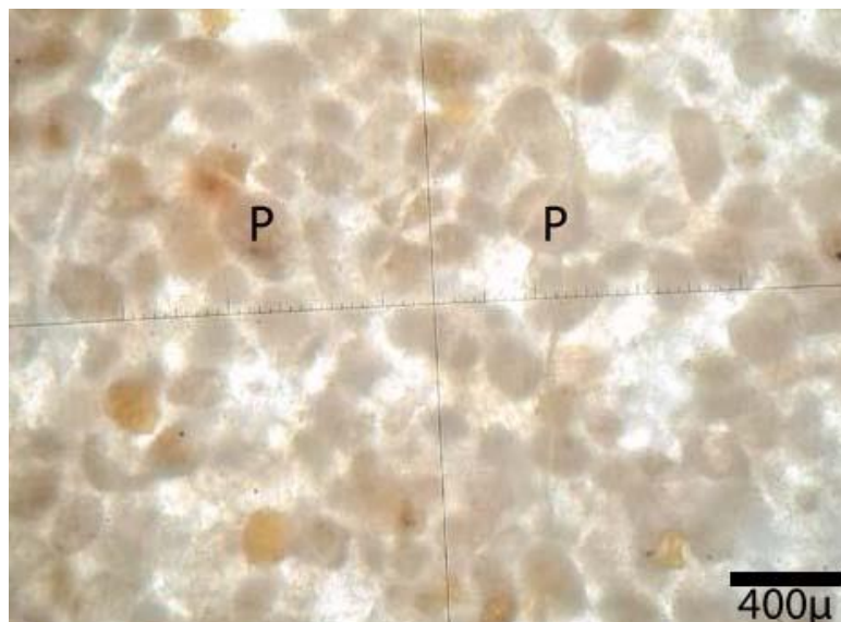
Figure 25: Grainstone (Pelsparite) à pelletoïdes (P) de taille variable.
