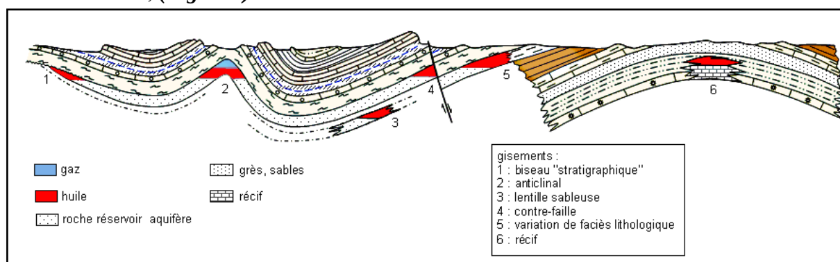
Fig. 102 : Coupe schématique de pièges stratigraphiques et structuraux
