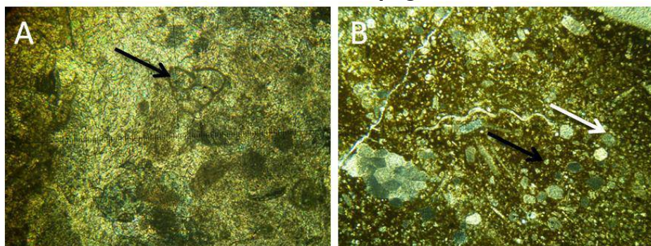
Mph.2: Microfaciès MO6 : packestone, biomicrite à dasycladacées, lamellibranches et crinoïdes. A : (flèche noire), Textularia, B : (flèche blanche) grains de quartz, (flèche noire), grains de dolomite (Y2, LN, X 2,5)
