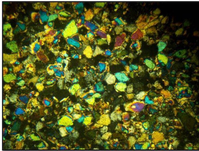
Mph.2: Microfaciès GR2, Grès à ciment argileux (BC 1.1 LP, X 2,5(X1,25))
