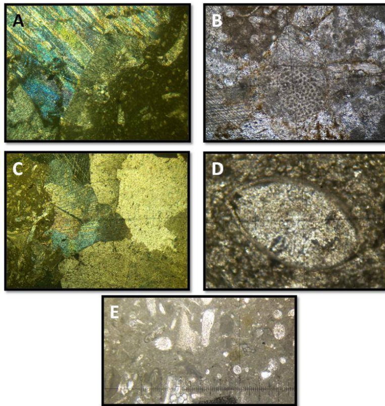
Mph2 : Ciments calcitiques : A, C : ciment drusique sparitique développé dans des vides, B : ciment drusique microsparitique et syntaxique au niveau d'une plaque de crinoïde dans le coin inférieur gauche, D : ciment drusique microsparitique développé au cœur d'un ostracode et E : ciment micritique
