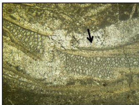
Mph.8 : Microfaciès EXP2, recristallisation de la micrite en microsparite en contact des tests d'huître (flèche noire) (E4, LN, X 2,5 (X1, 25))
