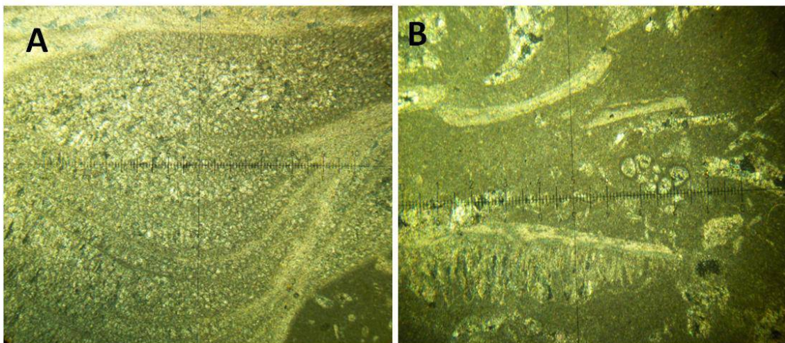
Mph.1: Microfaciès EXP6 : pack-rudstone à huîtres et rudistes, A : test d'huître avec les deux couches, lamellaire et vésiculaire, B : fragments de rudistes dans une biomicrite (BC 1.6, LN, X 2,5 (X1, 25))
