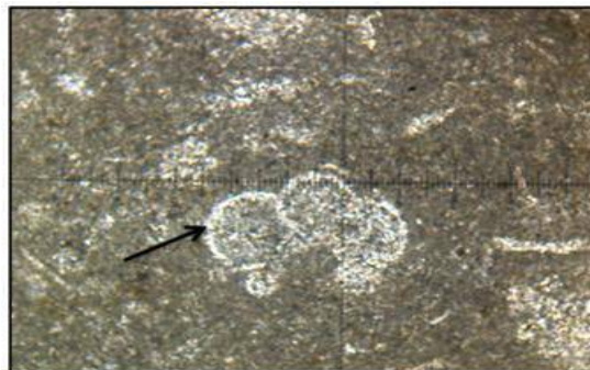
Mph.3 : Microfaciès EXD4 : wackestone, biomicrite à foraminifères planctoniques et ostracode. Hedbergella .sp (flèches noire) (E6, LN, X 10 (X1, 25))
