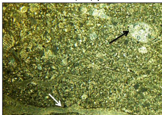
Mph.3: Microfaciès MO7 : packestone, biomicrite à rudistes et ostracodes. Flèche noire : Ostracode, flèche blanche : rudistes (Y3, LN, X 2,5 (X1, 25))
