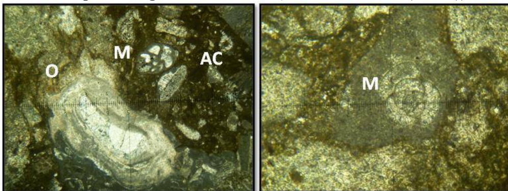
Mph.2: Microfaciès CG2, microconglomérats à ciments argilo-carbonaté oxydé. M : miliolles, O : oncoïdes, AC : ciment argilo-carbonaté oxydé (BC 1.5 LN, X 2,5 (X1, 25))
