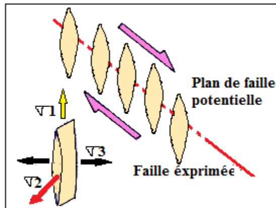
Fig.72: Fentes de tension en échelon le long d'une faille potentielle avec un détail montrant la géométrie de l'ouverture par rapport aux contraintes
