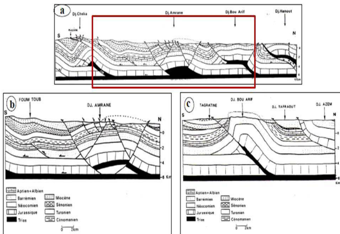
Fig. 86 : Coupes interprétatives des structures plissées du bassin de Timgad, montrant un chevauchement vers le sud. a : front du chevauchement; b : anticlinaux de Foug Toub et Dj. Amrane; c : Anticlinal du Dj. Bou Arif et Synclinal de Tagratine (Ghandriche, 1991).
