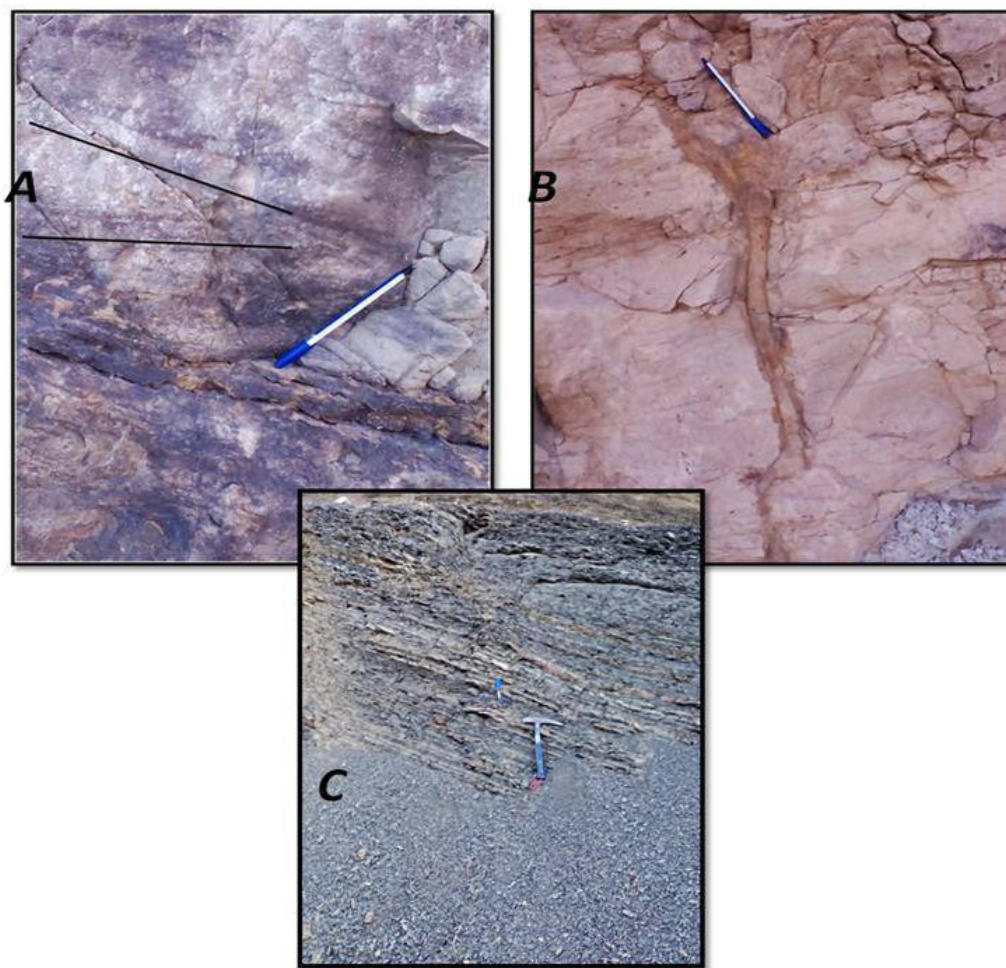
Fig. 49: A : Litage entrecroisé dans les grés du Membre 4B de la formation F4 B : Terrier vertical dans les marnes du Membre 4A de la F4 C : Débit en frites des marnes du Membre 4B de la formation F4
