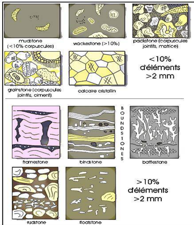
Fig. 61: Classification des roches calcaires selon Dunham (1962) et Embry & Klovan (1972).
