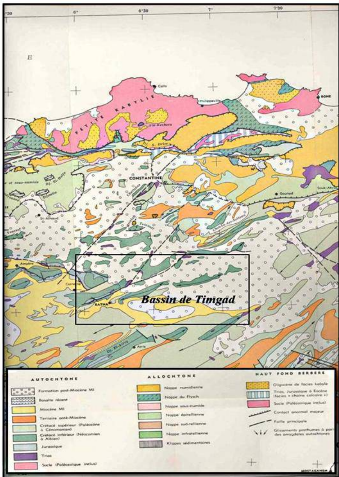
Fig. 10 : Carte géologique montrant les différentes formations de l'Avant pays méridional de la chaîne des Maghrébides
