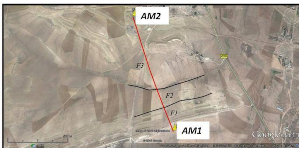
Fig. 35: Image satellitaire représentant les formations lithologiques traversées par la coupe de Guabel Amrane
