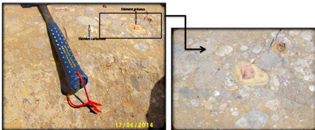
Fig. 26 : Photo représentant le banc conglomératique avec un détail des différents éléments
