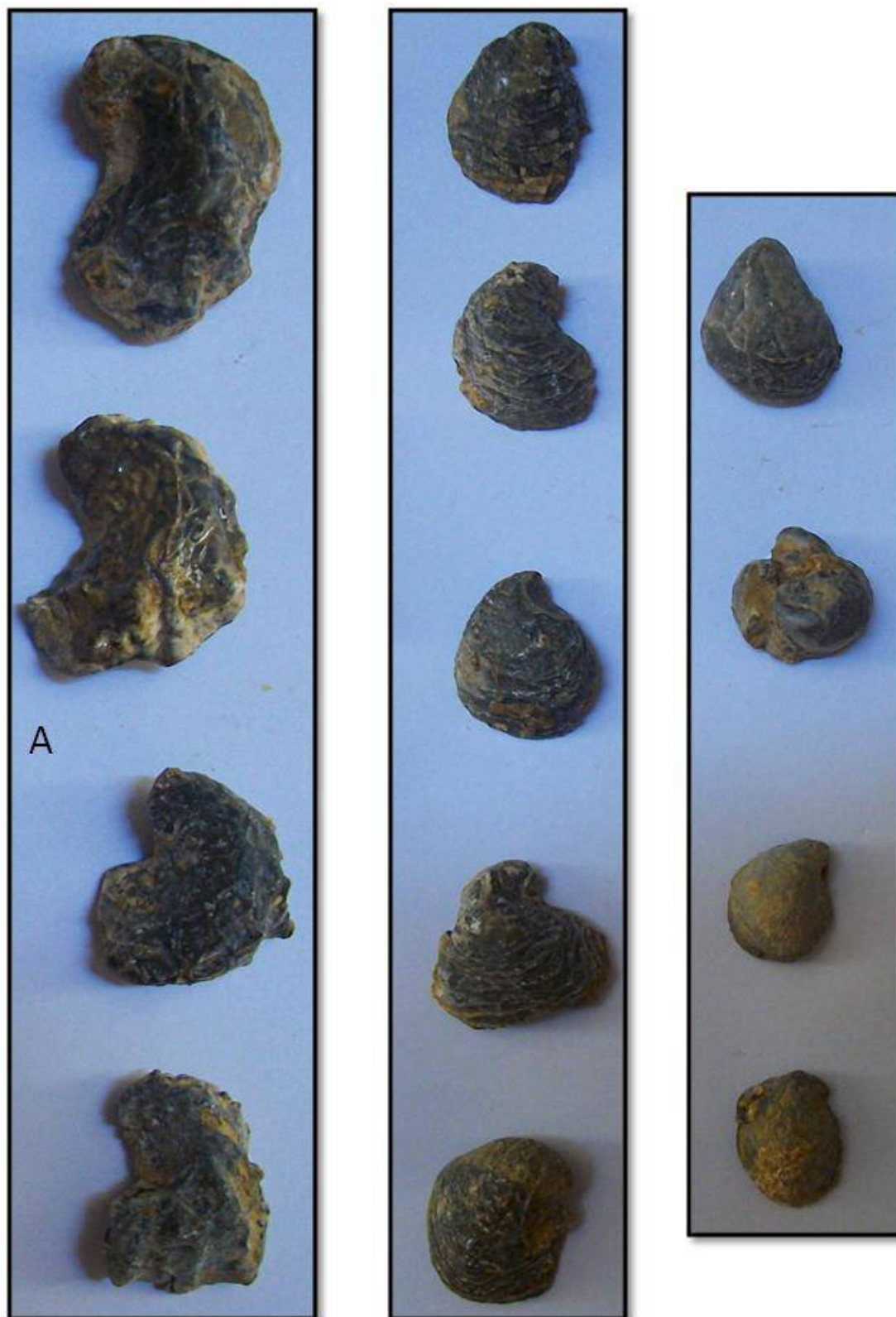
PH1 : Exogyra, Lamarck, 1801, récoltés dans les marnes du Cénomanién de Dj. Amrane, X1. A : Ilymatogyra (Afrogyra) Africana.
