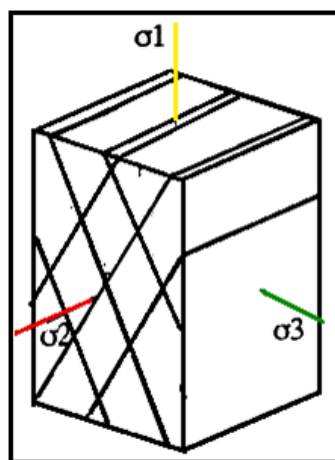
Fig. 73 : Système de diaclases
