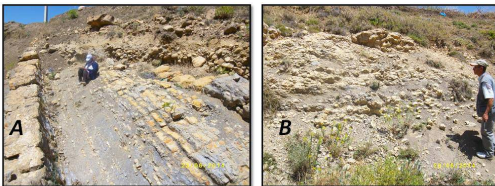
Fig. 44: A : Faciès marno-calcaire du membre 1A de la F1;
