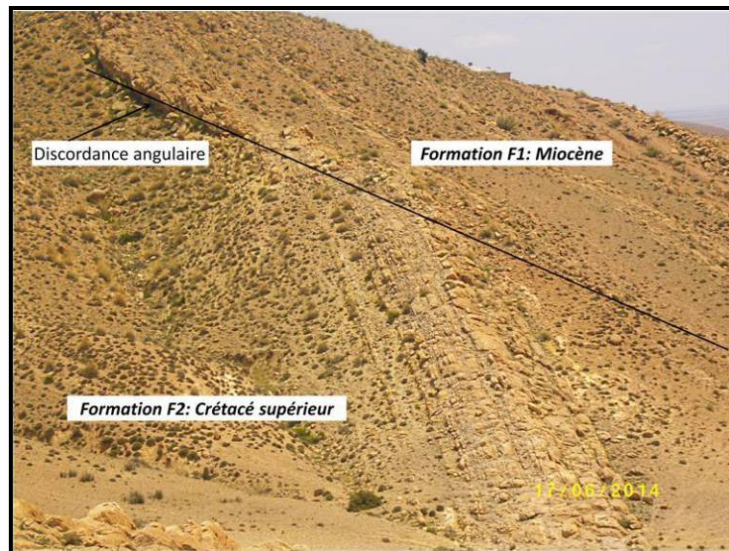
Fig. 30 : Discordance angulaire de Tortonien sur le Coniacien
