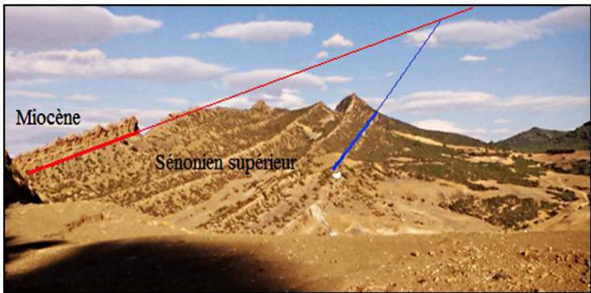
Fig. 47: Photo panoramique montrant la discordance angulaire du Miocène sur les formations du Sénonien supérieur (région de Yabous). (Les traits rouge et bleu révèlent les pendages des couches)
