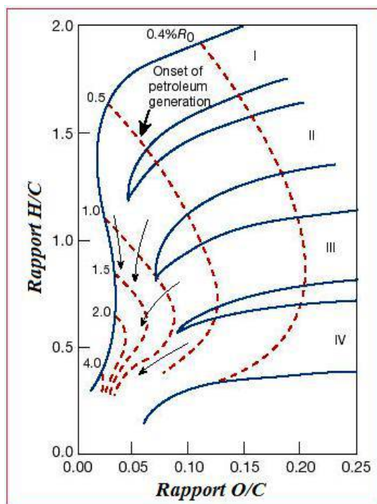
Fig. 97 : Diagramme de Van Krevelen indiquant la composition élémentaire des quatre principaux types de kérogène
