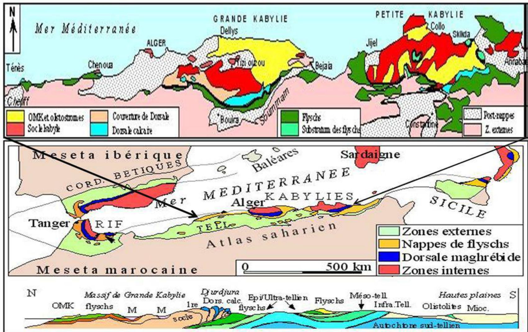
Fig. 7 : Carte structurale schématique de la chaîne Maghrébides montrant la disposition des zones internes et externes; d'après Durand Delga et Fontbonté (1980)
