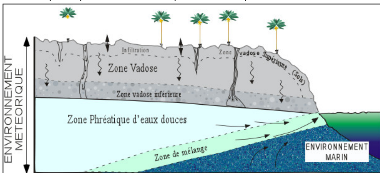
Fig.64 : Modèle conceptuel des principaux environnements diagenétiques (Moore, 2001)
