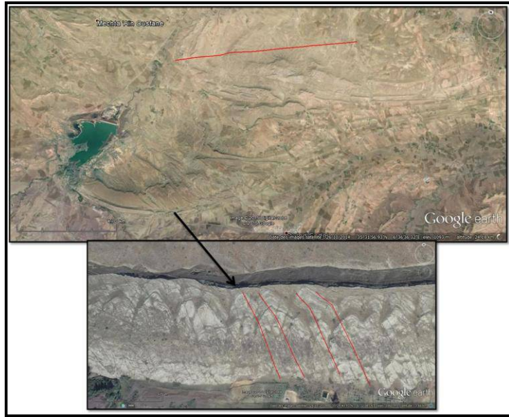
Fig. 83 : Vue 3D de la structure de Dj. Amrane sur image satellite de Google Earth
