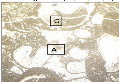
Mph.4: Microfaciès EXP5, wackestone, biomicrite à algues et annélides, A : Annélides, G : Gastéropode, (KM 1.6-1.9 LN, X 5)
