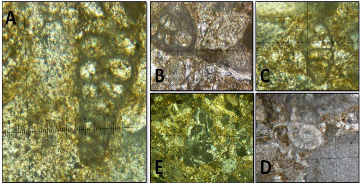
Mph.1: Microfaciès IN2, grainstone, intrabiosparite à foraminifères benthiques et bryozoaires IN3: grainstone, Intrabiosparite à foraminifères benthiques et bryozoaires
