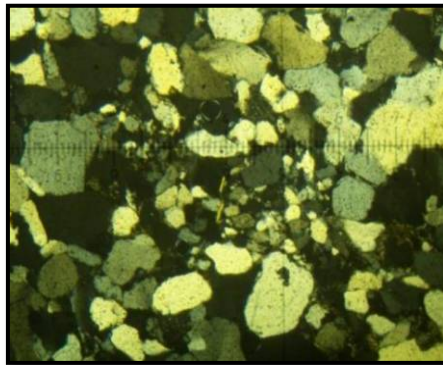
Mph.10: Microfaciès GR3, Grès à ciment argileux au centre de la microphoto, un terrier rempli de grains plus petits que ceux de la roche avec ici un ciment carbonaté (BC 1.2 LP, X 2,5(X1, 25))
