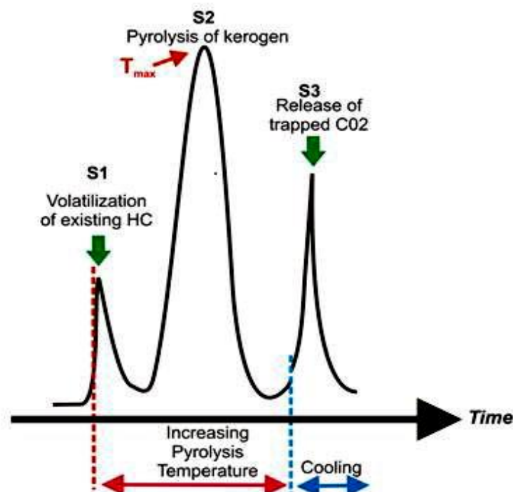
Fig. 99 : Pyrolyse programmée, exemple d'un pyroprogramme
