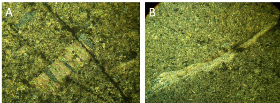
Mph.1: Microfaciès MO5 : wackestone, biomicrosparite à lamellibranches A : section prismatique de lamellibranche dans un calcaire recristallisé, B : fragment de rudiste (Y1, LN, X 2,5 (X2))
