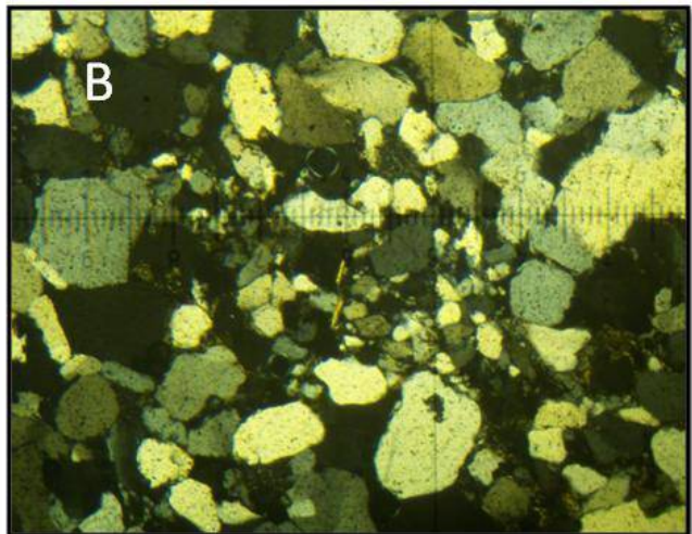
Mph.3: Microfaciès GR3, Grès à ciment argileux ? A : ciment argileux, B : au centre de la microphoto, un terrier rempli de grains plus petits que ceux de la roche avec ici un ciment carbonaté (BC 1.2 LP, X 2,5(X1, 25))
