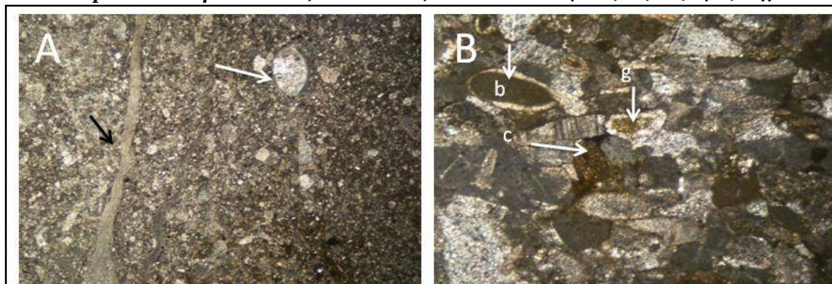
Mph. 3: Microfaciès MO3 : packestone, biomicrite à lamellibranches, dasycladacées et échinides. A : Rudiste (flèche noire), Ostracode (flèche blanche) ; B : b : bahamite, g : glauconie et c : section de crinoïdes (Ech8, LN, X 2,5 (X1, 25))
