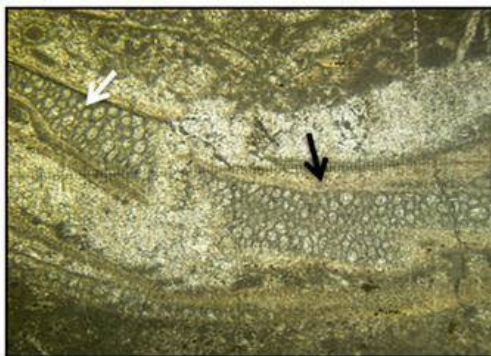
Mph.1: Microfaciès EXP2, packstone, biomicrite à grand débris d'huitres ;test d'huitre avec les deux couches, lamellaire (flèche noire) et vésiculaire (flèche blanche) (E4, LN, X2,5 (X1, 5))
