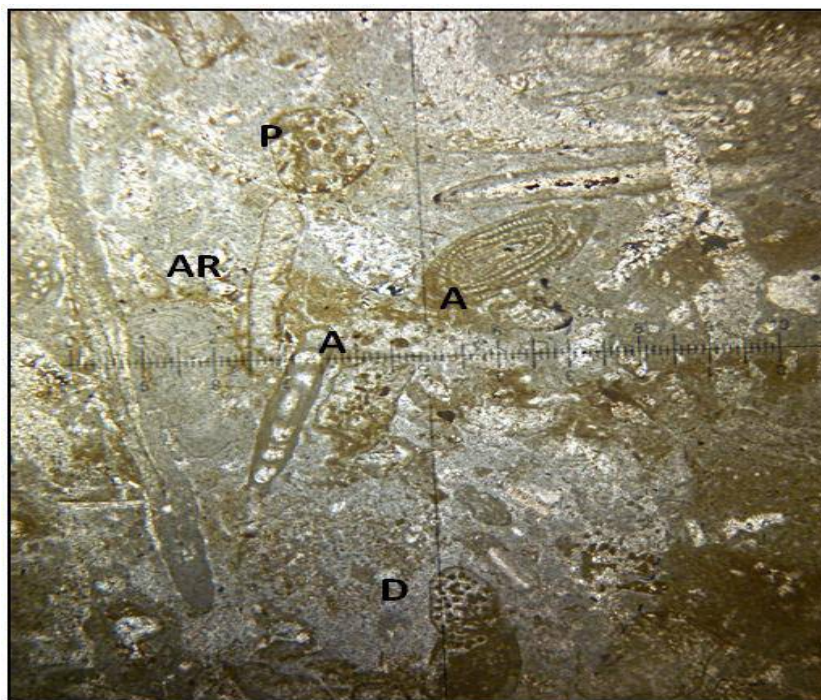
Mph.1: Microfaciès MO1 : packestone, biomicrite à algues. A : Alvéolina, D : Dasycladacées, AR : Algues rouges et P : Pellets (A2b, LN, X 2,5 (X1, 25))
