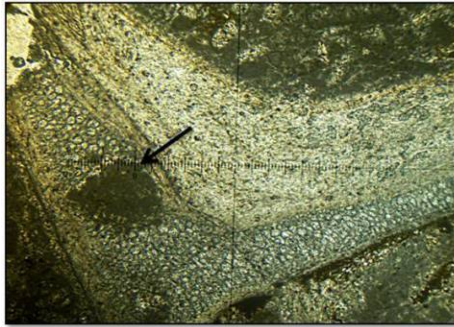
Mph.9: Microfaciès EXP4, perforation d'un test d'huître puis remplissage par de la micrite (flèche noire) (A2, LN, X 2,5 (X1, 25))
