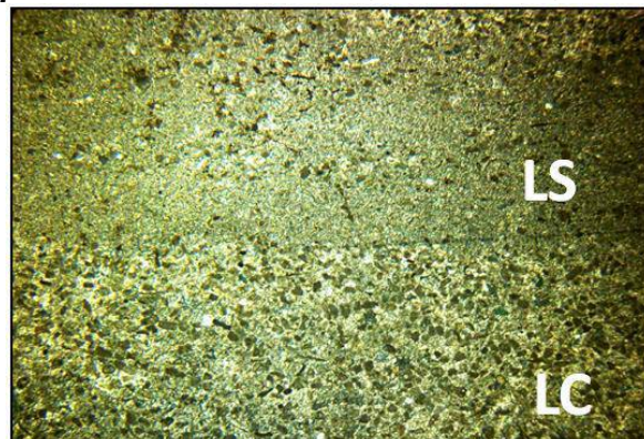
Mph4: Microfaciès MO8 : tempestites proximales LS : lamine sombre, LC : lamine claire. (YA, LN, X 2,5)
