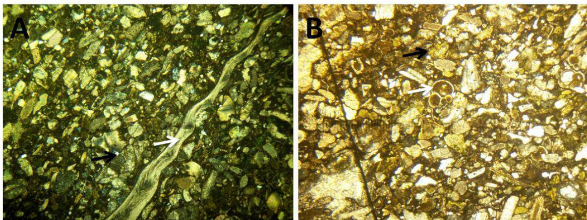
Mph.3: Microfaciès EXP8 : packestone, biomicrite à foraminifères planctoniques, benthiques et rudistes A : flèche noire : quartz, flèche blanche : rudistes ? (BC 1.3, LP, X 2,5 (X1, 25)) B : flèche noire : glauconie, flèche blanche : globigérines (BC 1.3, LN, X 2,5 (X1, 25))
