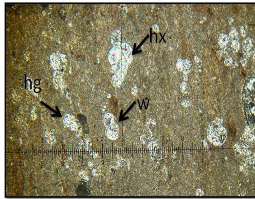
Mph.1: Microfaciès EXD1, wackestone, biomicrite à foraminifères planctoniques. w: Whiteinella helvetica ; hx: Heterohelix globulosa hg: Hedbergella . sp (E1, LN, X10 (X1,25))
