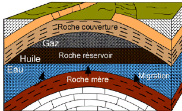
Fig. 100 : Modèle d'un système pétrolier
