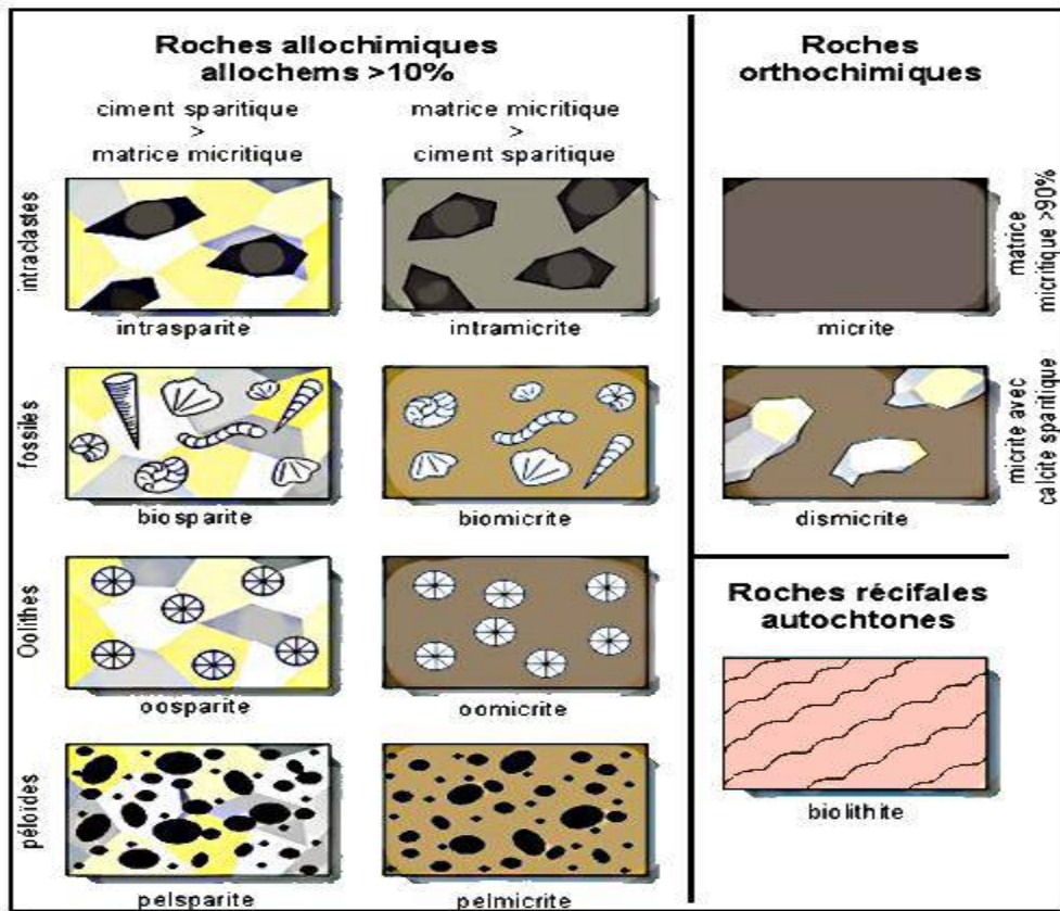
Fig. 60: Classification des roches calcaires selon Folk (1959).
