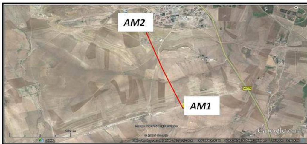
Fig. 34: Image satellitaire représentant la coupe de Guabel Amrane dans son cadre géographique
