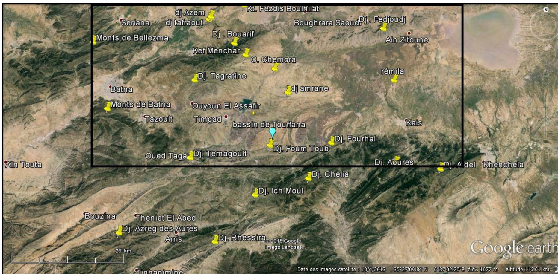
Fig. 3 : Toponymie de la région d'étude et ses environs
