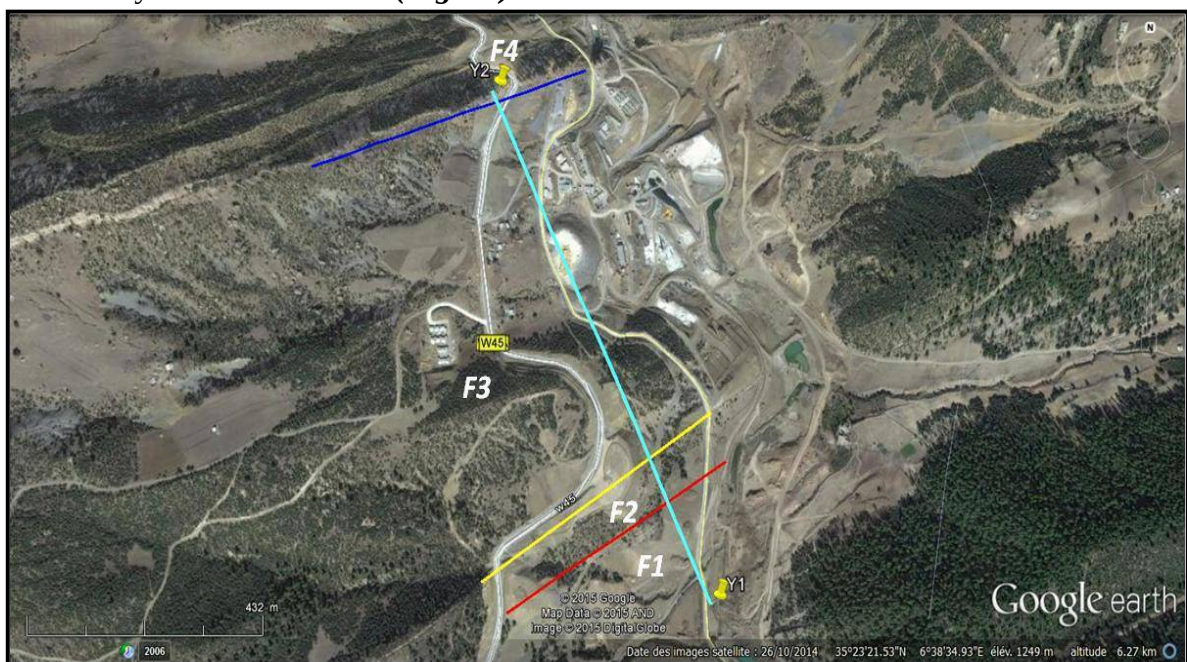
Fig. 43: Image satellitaire montrant les formations lithologiques traversées par la coupe de Yabous
