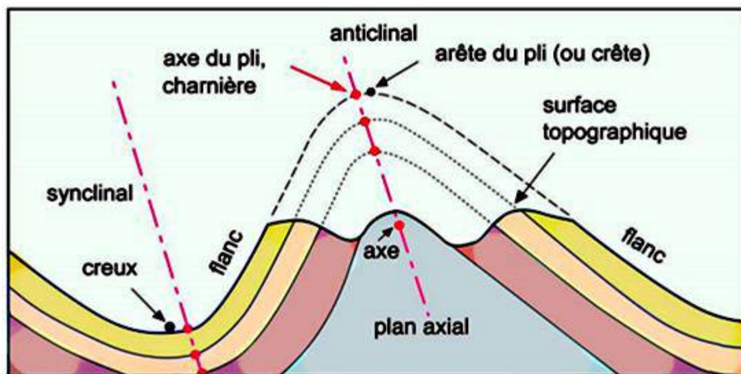
Fig. 75 : Structure d'un pli
