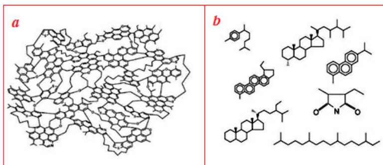
Fig. 96 : Fractions d'hydrocarbures : (a) Modèle structural d'un kérogène (b) Exemples de molécules organiques typiques de la fraction extractible. Béhar & Vandenbroucke (1986).
