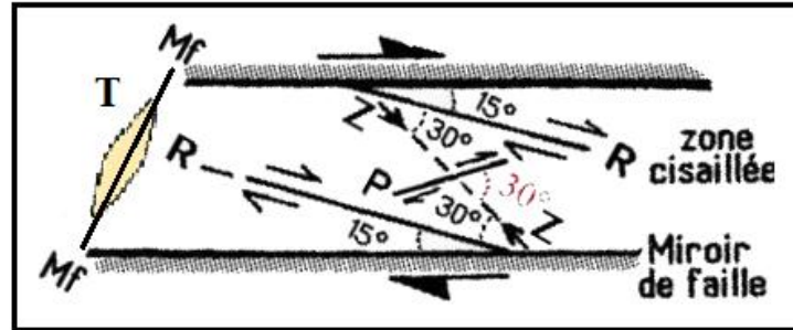
Fig. 74 : Système de Riedel
