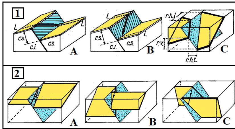
Fig. 70 : Rejets des failles
