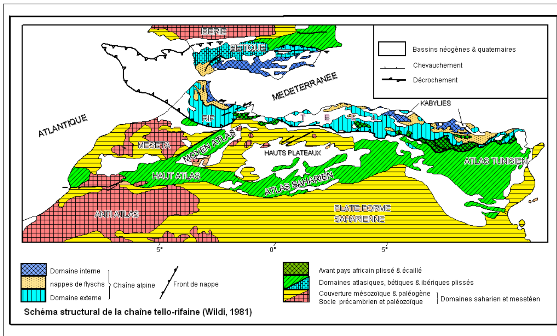
Fig. 6 : Schéma structural de la chaîne des Maghrébides
