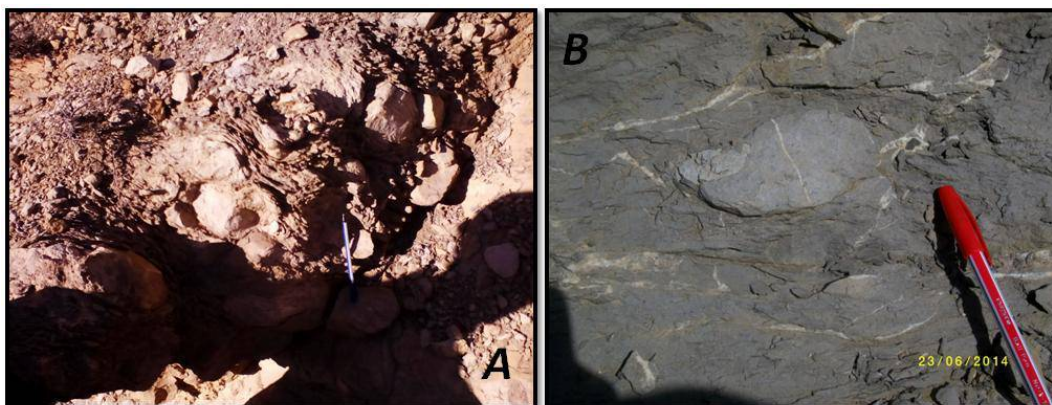
Fig. 46 : A : Enveloppe marneuse autour de nodule calcaire B : Nodule calcaire argileux enveloppé de marne membre 1B de la F1
