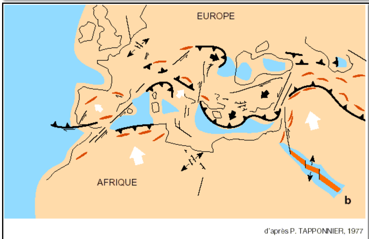
Fig.16 : Enchaînement géodynamique à l'Oligocène (a) et au Quaternaire (b).
