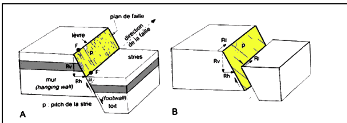
Fig. 68 : Schéma illustrant des failles verticales
