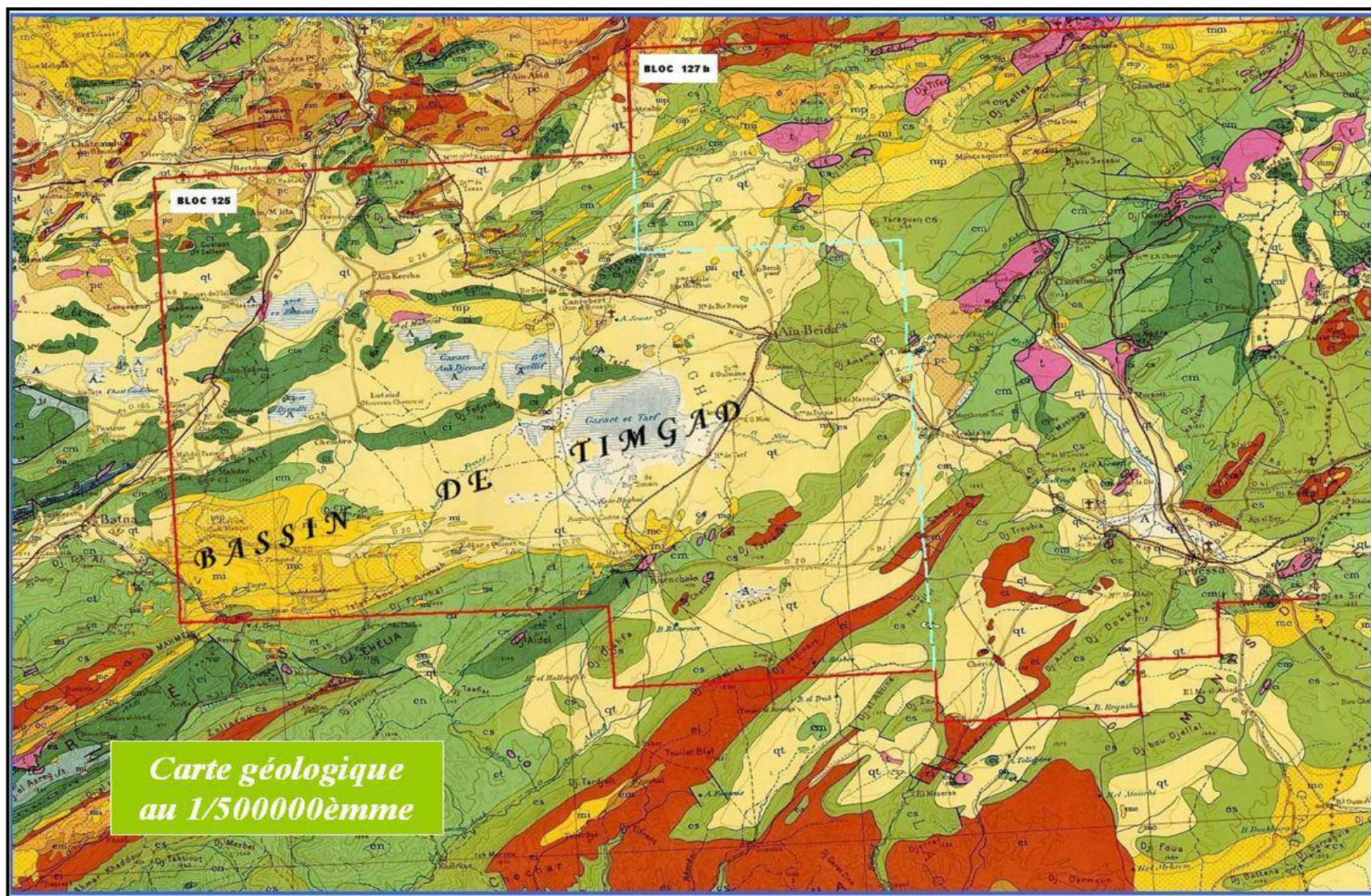
Fig. 11 : Carte géologique au 1/500000ème
