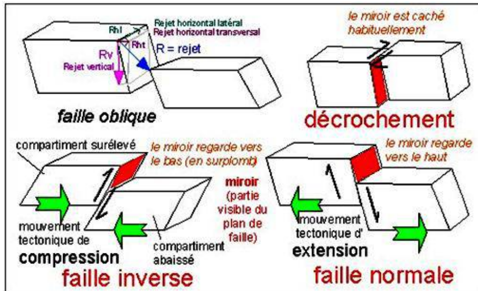
Fig. 69 : Types de Faïlles résultant des différents mouvements tectoniques
