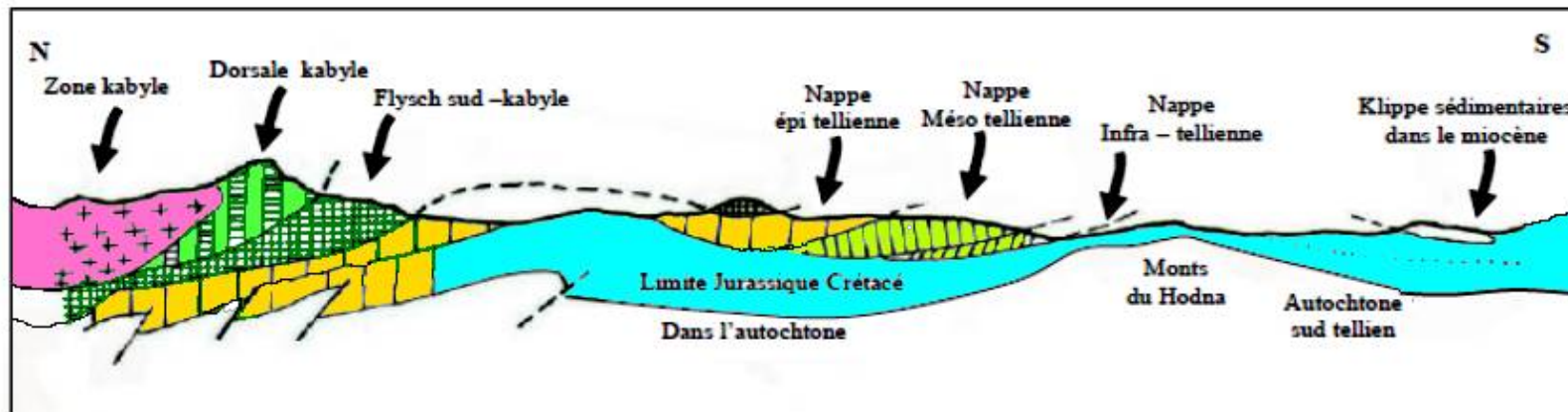
Fig.8 : Coupe géologique schématique illustrant les relations structurales entre les différentes unités de la chaîne alpine d'Algérie nord orientale (d'après M. Durand Delga, 1969)
