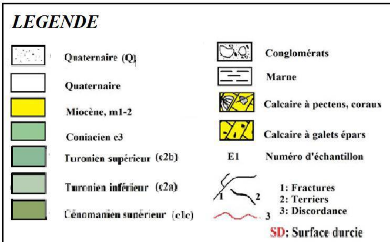
Fig. 32 : Légende des coupes géologiques
