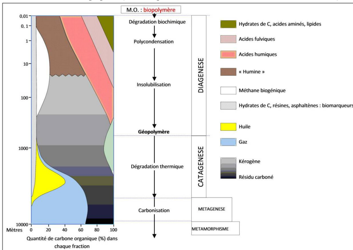
Fig. 98 : Évolution générale de la matière organique en fonction de la profondeur D'après Tissot & Welte et Edman & Surdam in Baudin, Tribovillard & Trichet
