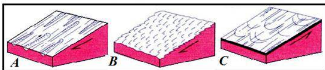
Fig.71: Microstructures de failles
