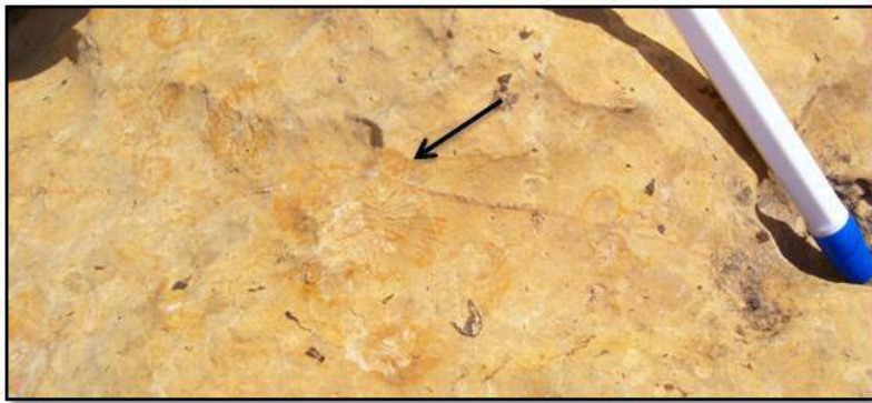
Fig. 37: Traces de coraux dans les calcaires du membre 3A
