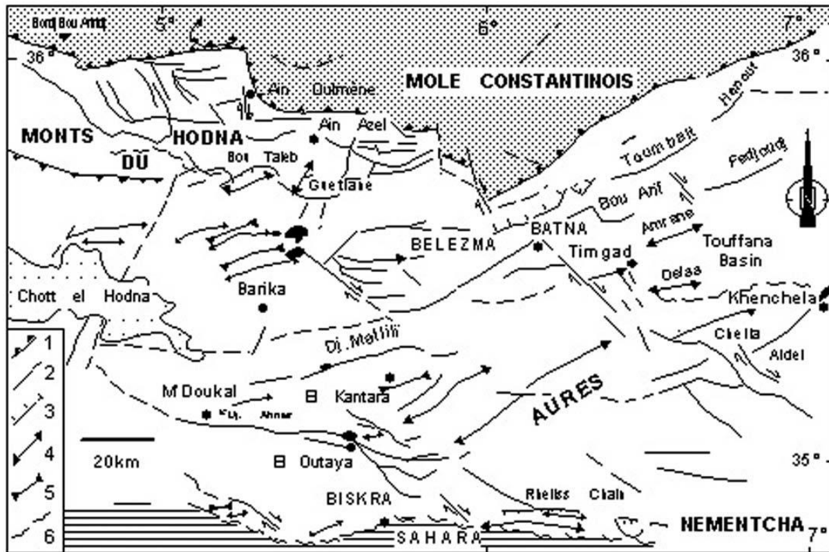
Fig. 17– Carte structurale des Monts du Hodna et des Aurès (Marmi et Guiraud, 2006) ; 1- front de nappe, 2- Faille, 3- Faille inverse, 4- Axe Anticlinal, 5- Axe Synclinal, 6- Flexure
