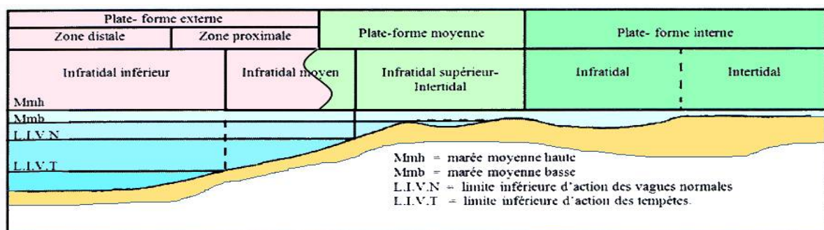
Fig.65 : Profil de la plate forme (Yahiaoui, 1990).
