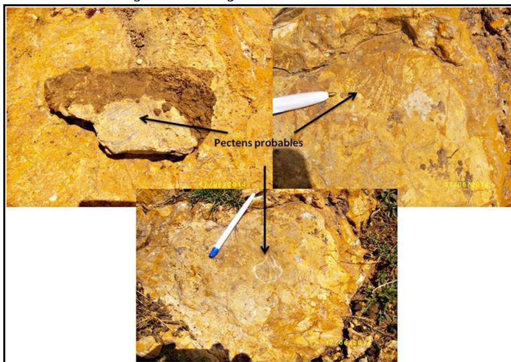
Fig. 28 : Pectens probables du membre 4D
