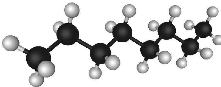
Fig. 95 : Schématisation de la formule brute de l'Octane
