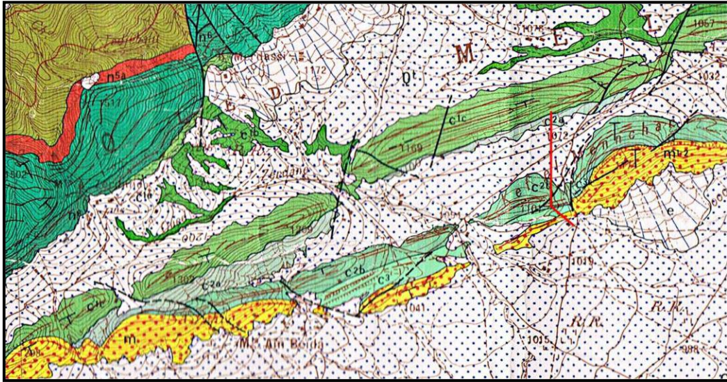
Fig. 29 : Tracé de la coupe sur un extrait de la carte géologique d'El Madher au 1/50000 ème
