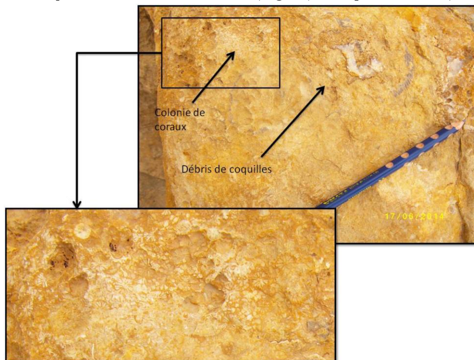
Fig. 24 : Débris de coquille et colonie de coraux dans le terme basal, membre 4A
