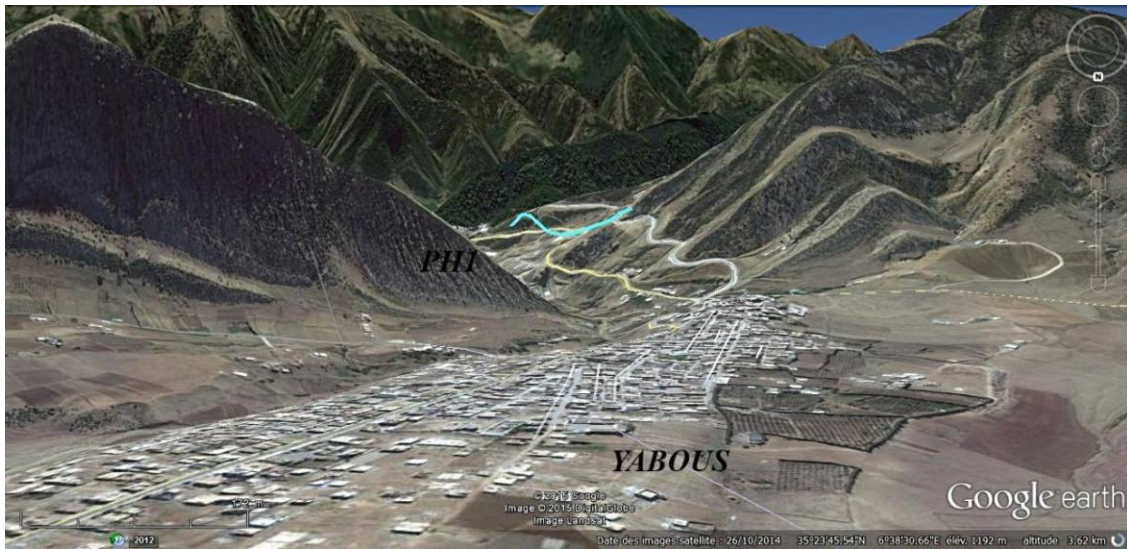
Fig. 42: Image satellitaire représentant la coupe de Yabous dans son cadre géographique
