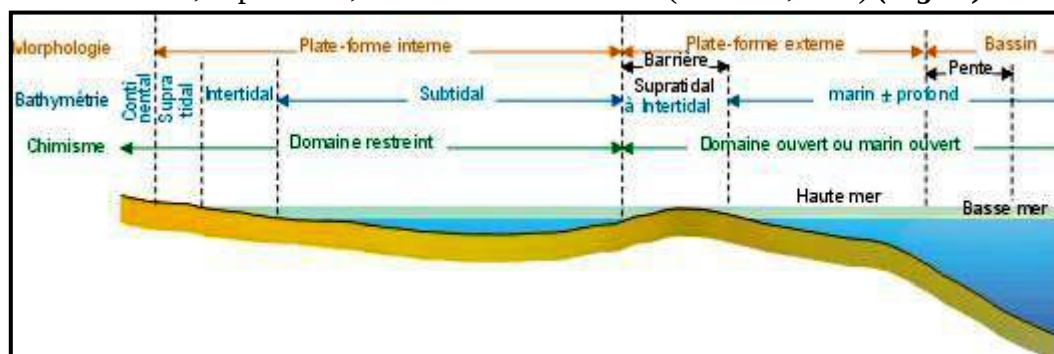
Fig.59 : Répartition des environnements sur une plate forme avec barrière (Turcker ,1995)
