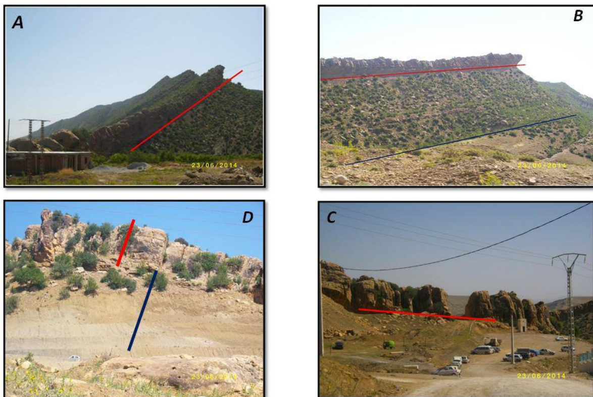
Fig. 48: Photos prises sous différents angles montrant la discordance angulaire du Miocène sur les formations du Sénonien supérieur (région de Yabous).
