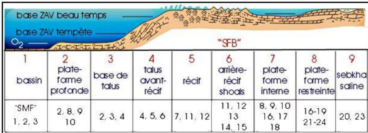
Fig.62: Microfaciès standards "SMF" et ceintures de faciès "SFB" de Wilson (1975) (hauteurs fortement exagérées).
