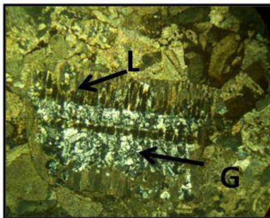
Mph.3: Microfaciès CG2, microconglomérats à ciments argilo-carbonaté, oxydé. G : gypse, L : lamellibranche, (BC 1.5 LN, X 2,5 (X1, 25))
