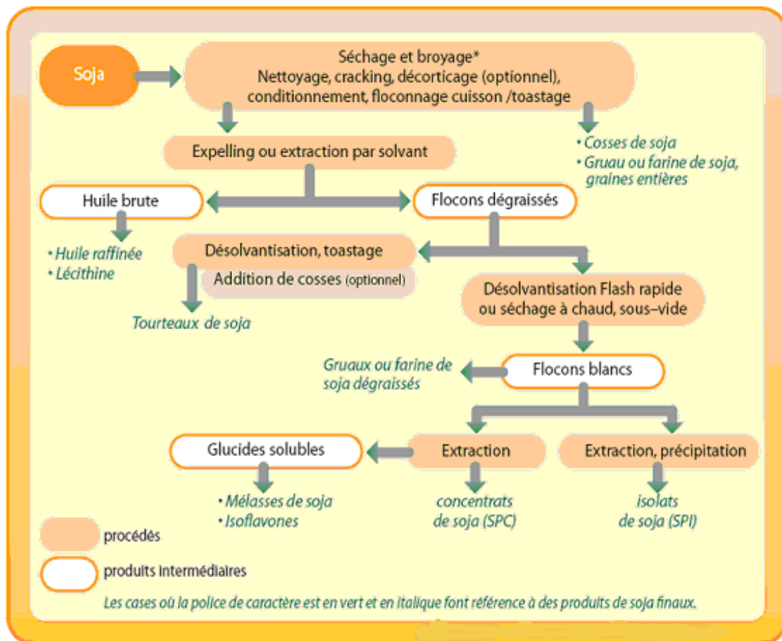
Figure n°07 : Représentation schématique de la fabrication des produits de soja, (NOPA, 1997).
